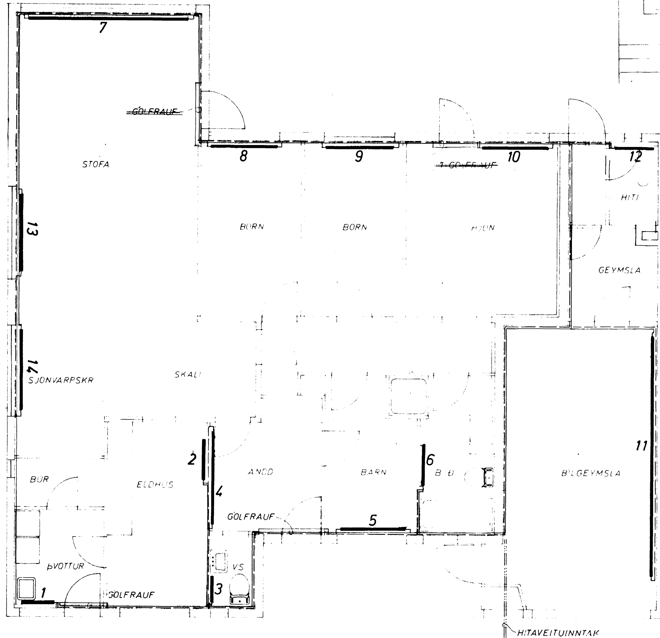
GRUNNMYND 1:50
