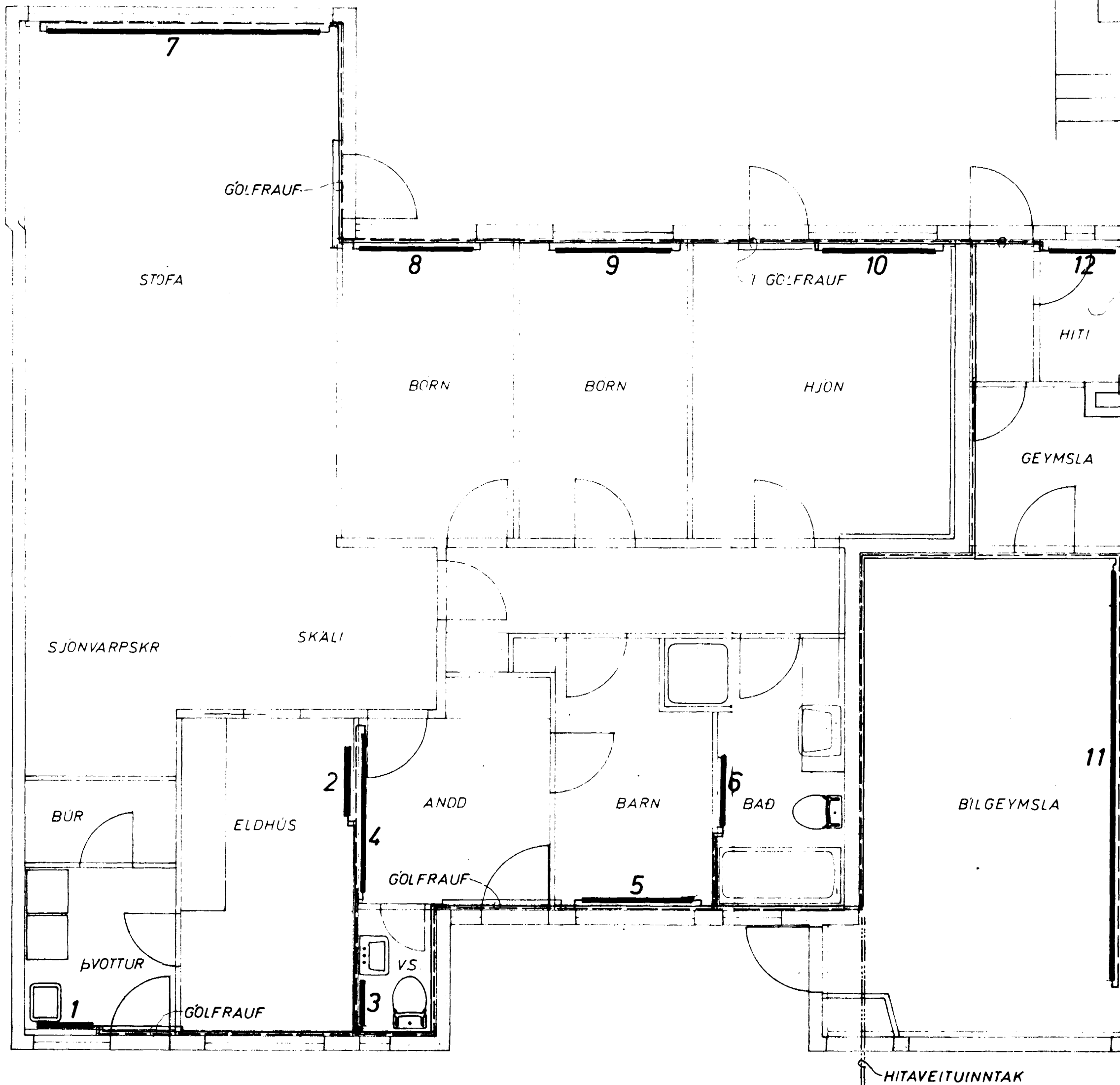
GRUNNMYND 1:50
