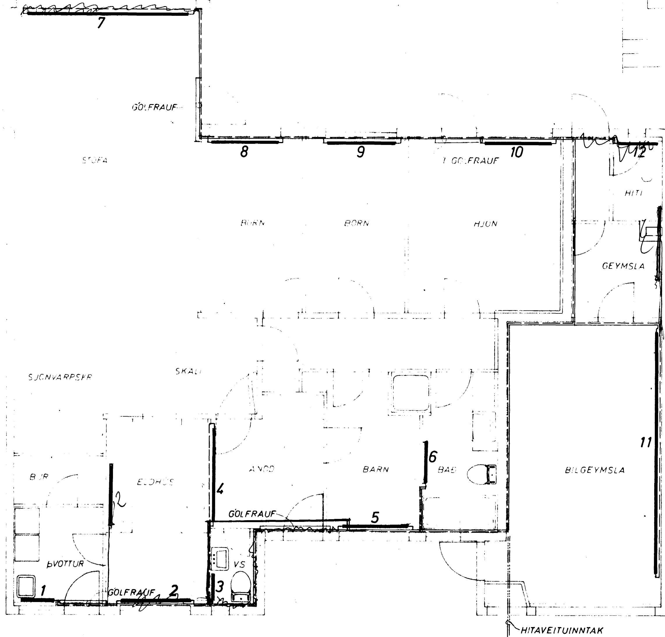
GRUNNMYND 1:50
