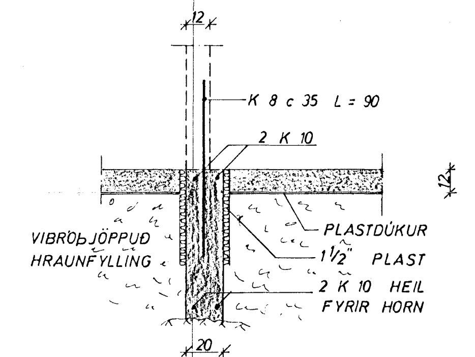
SNID 1 INNVEGG 1:20
