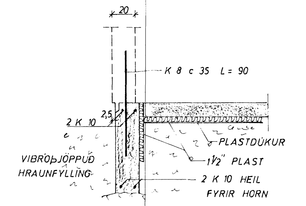
SNID 1 ÚTVEGG 1:20
