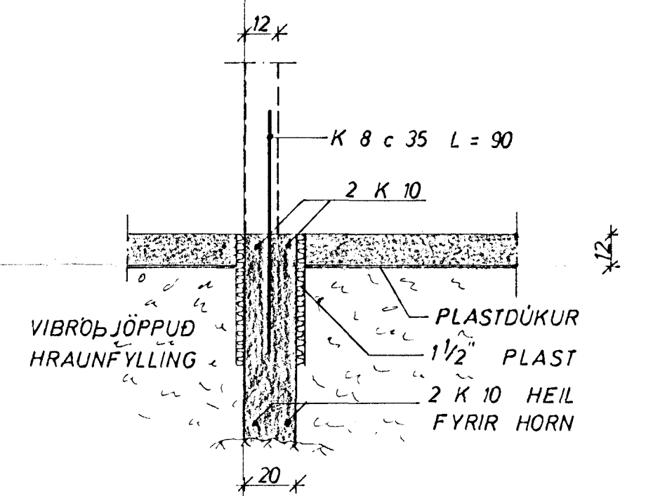
SNID 1 INNVEGG 1:20
