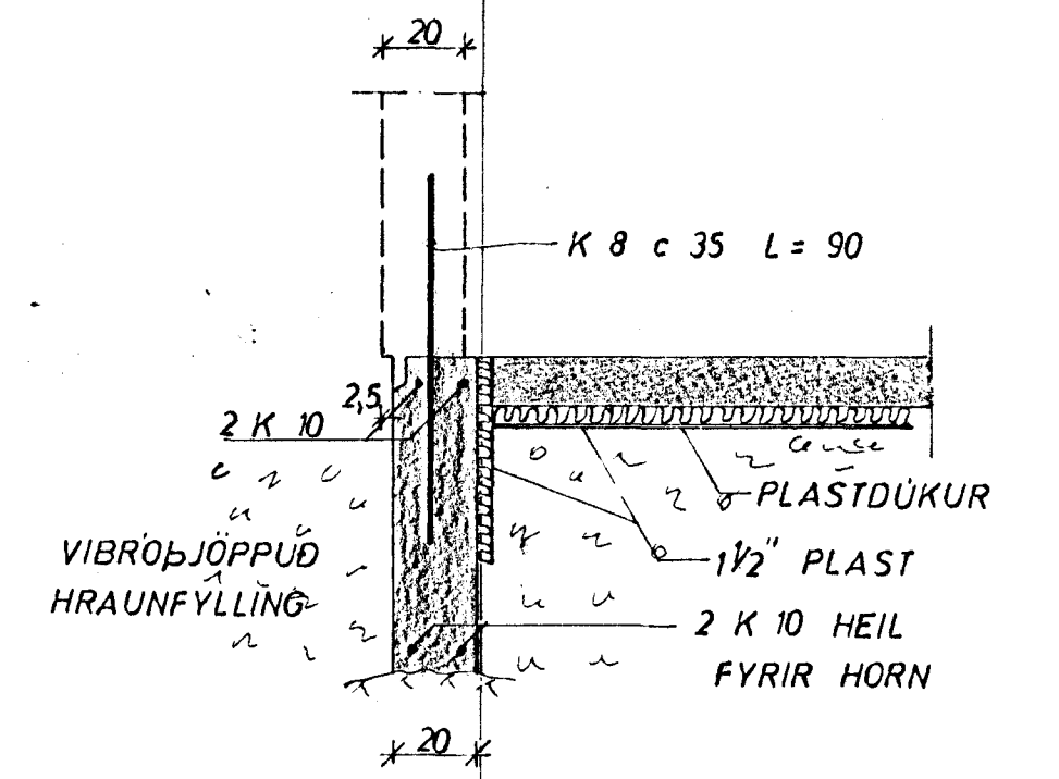
SNID 1 ÚTVEGG 1:20
