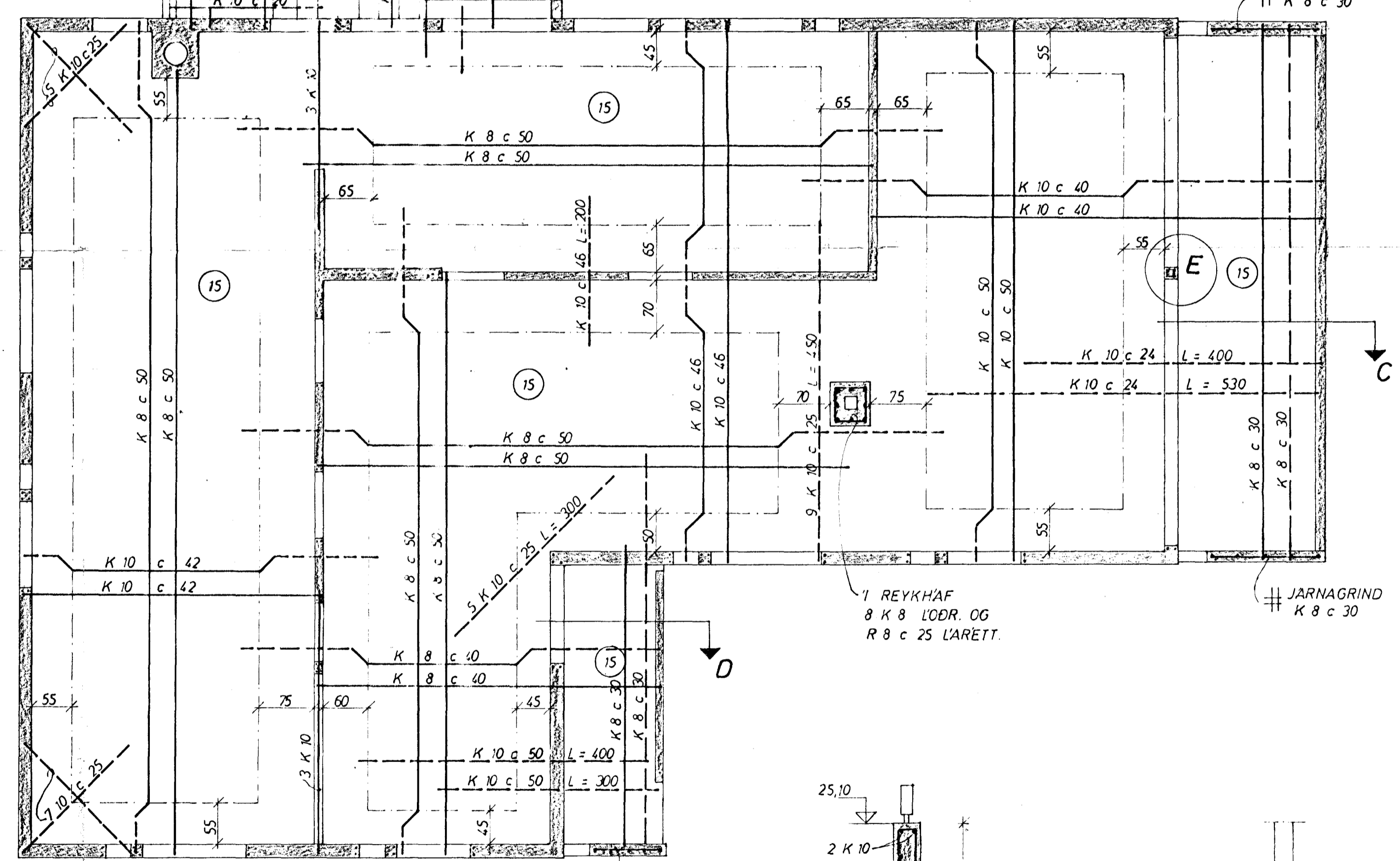
GRUNNMYND 1:50
