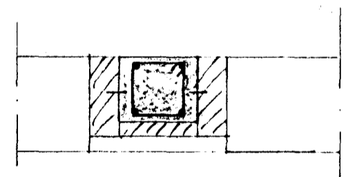
SÜLA E 1:10
