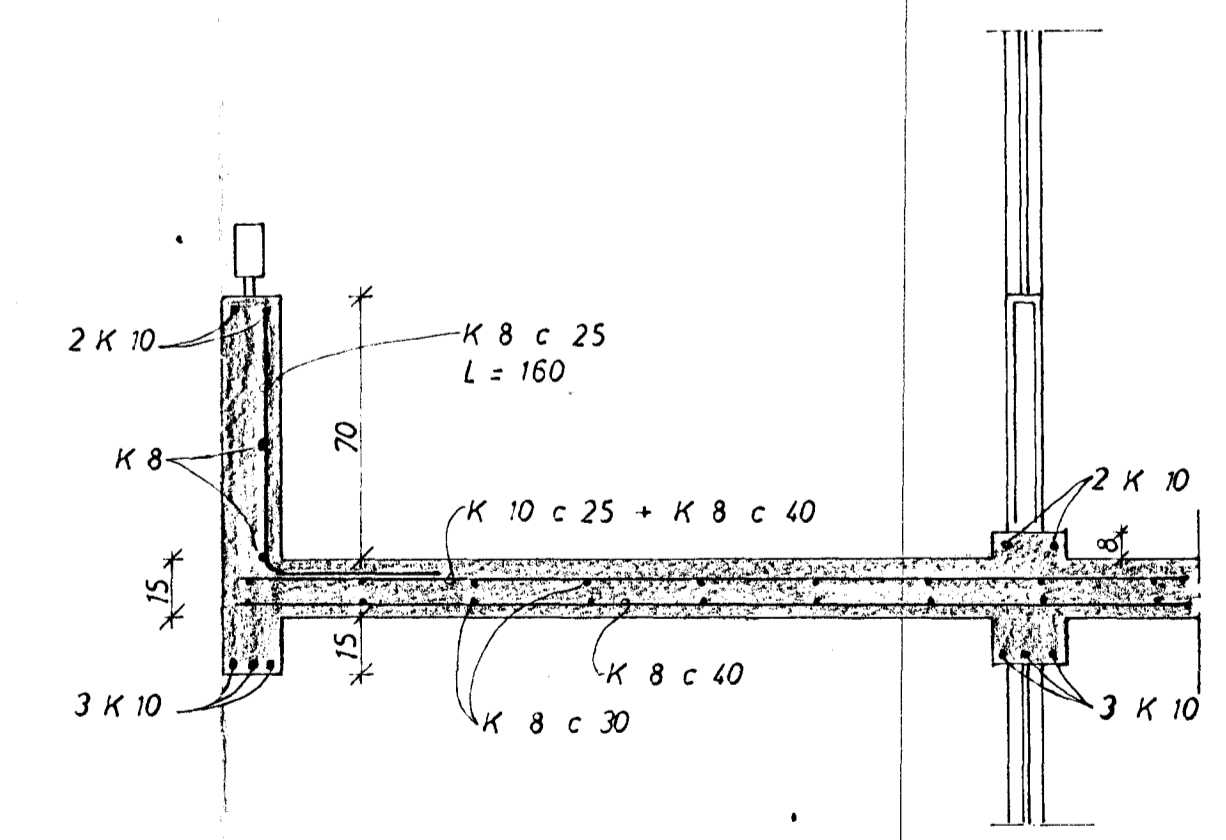
SNID D 1:20
