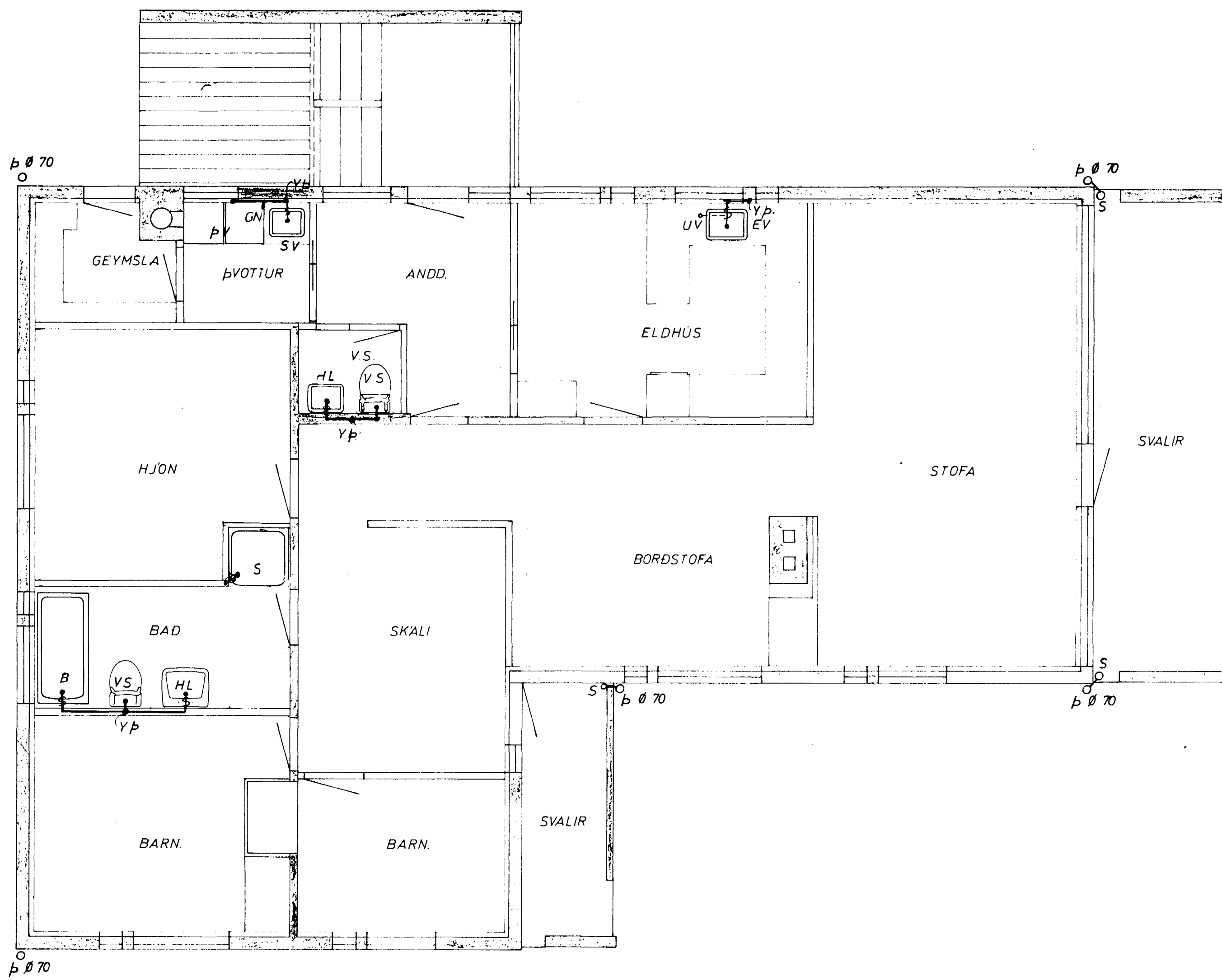
GRUNNMYND 1:50
