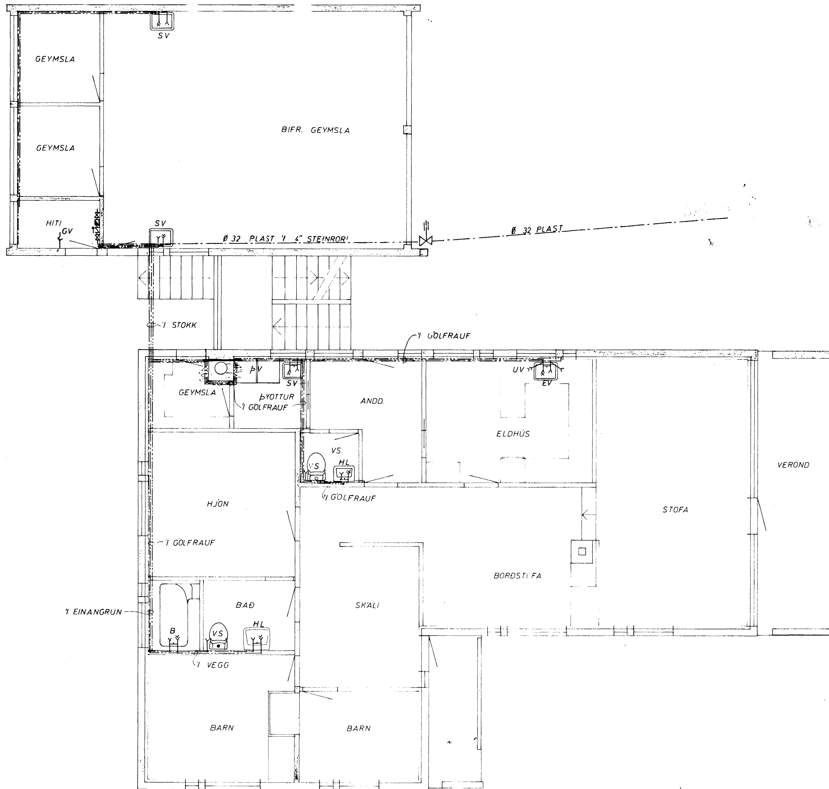
GRUNNMYND 1:50
