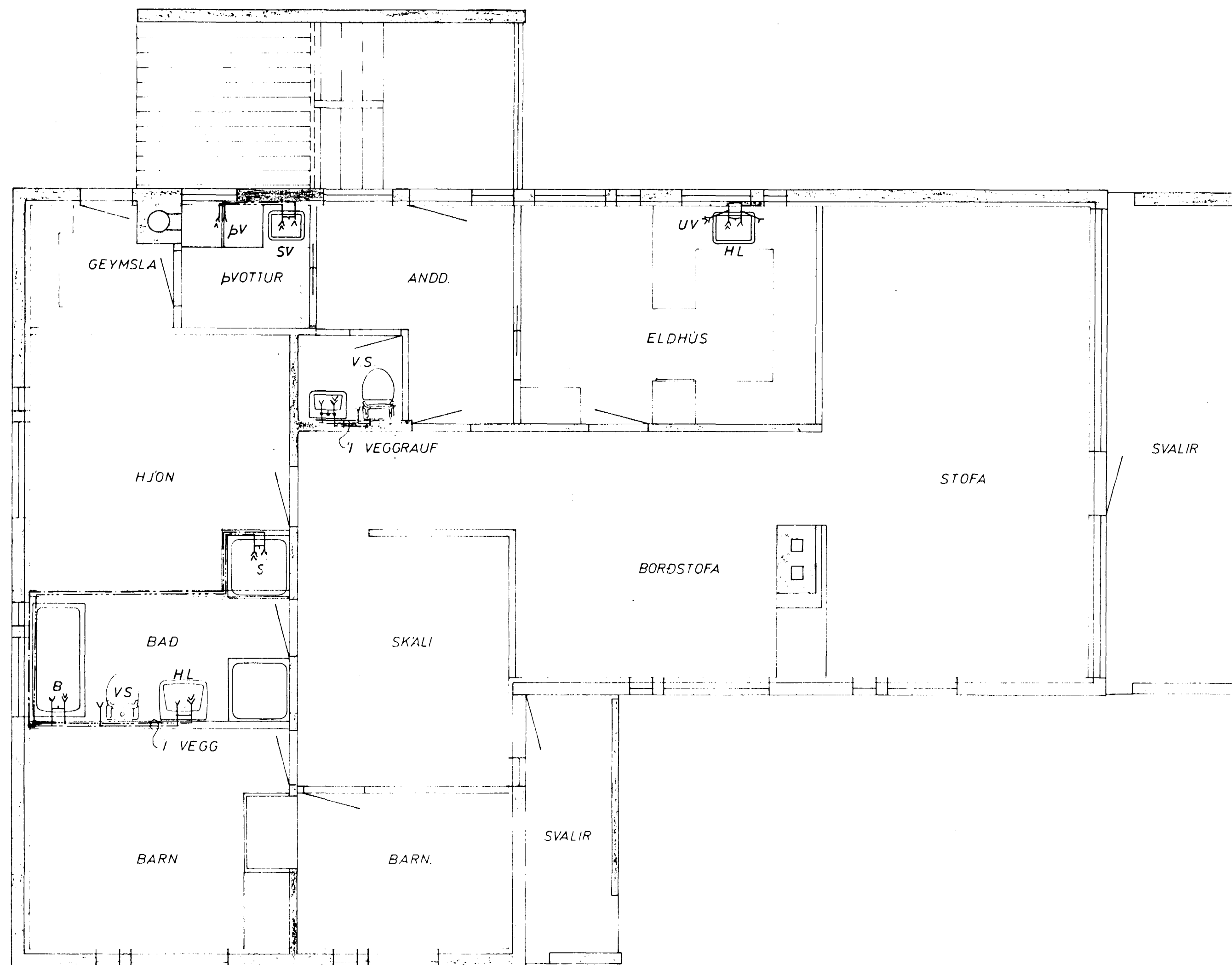
GRUNNMYND 1:50
