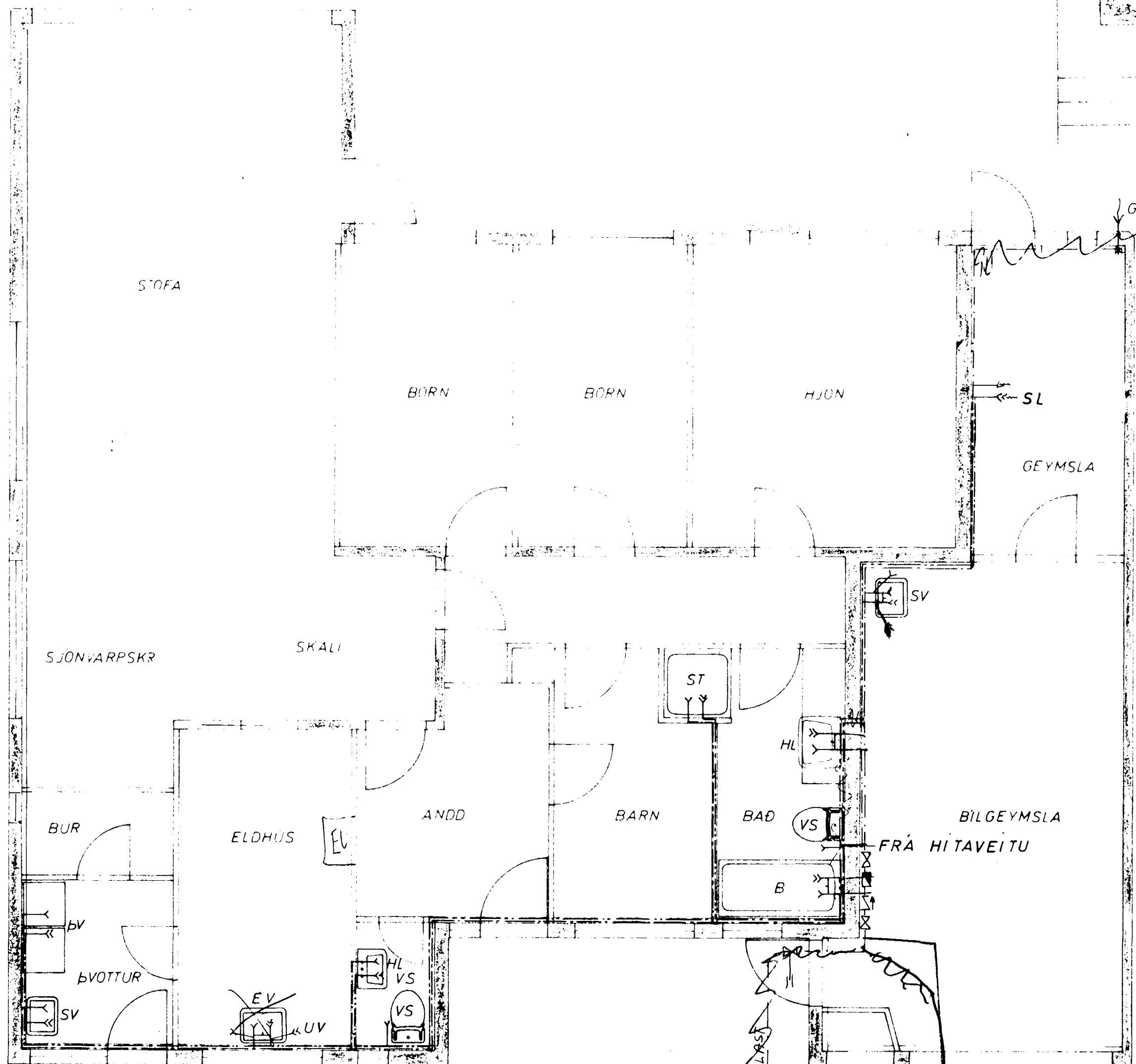
GRUNNMYND 1:50
