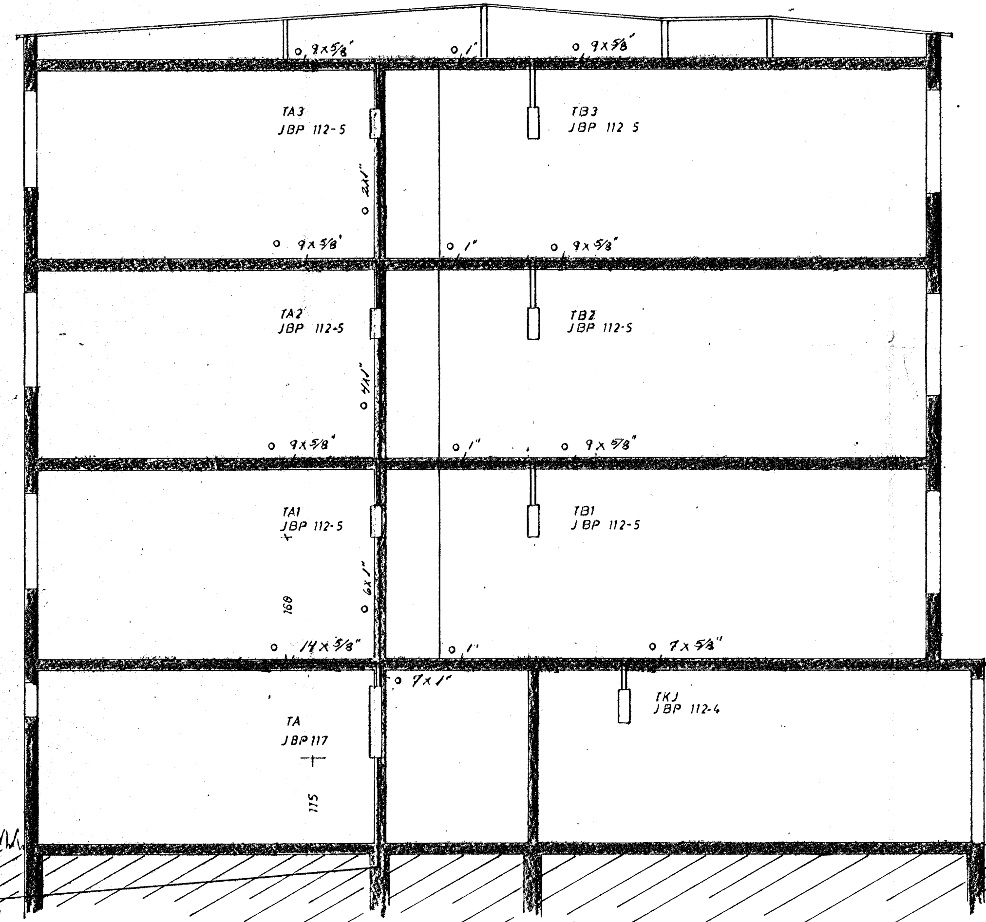
snid A-A
