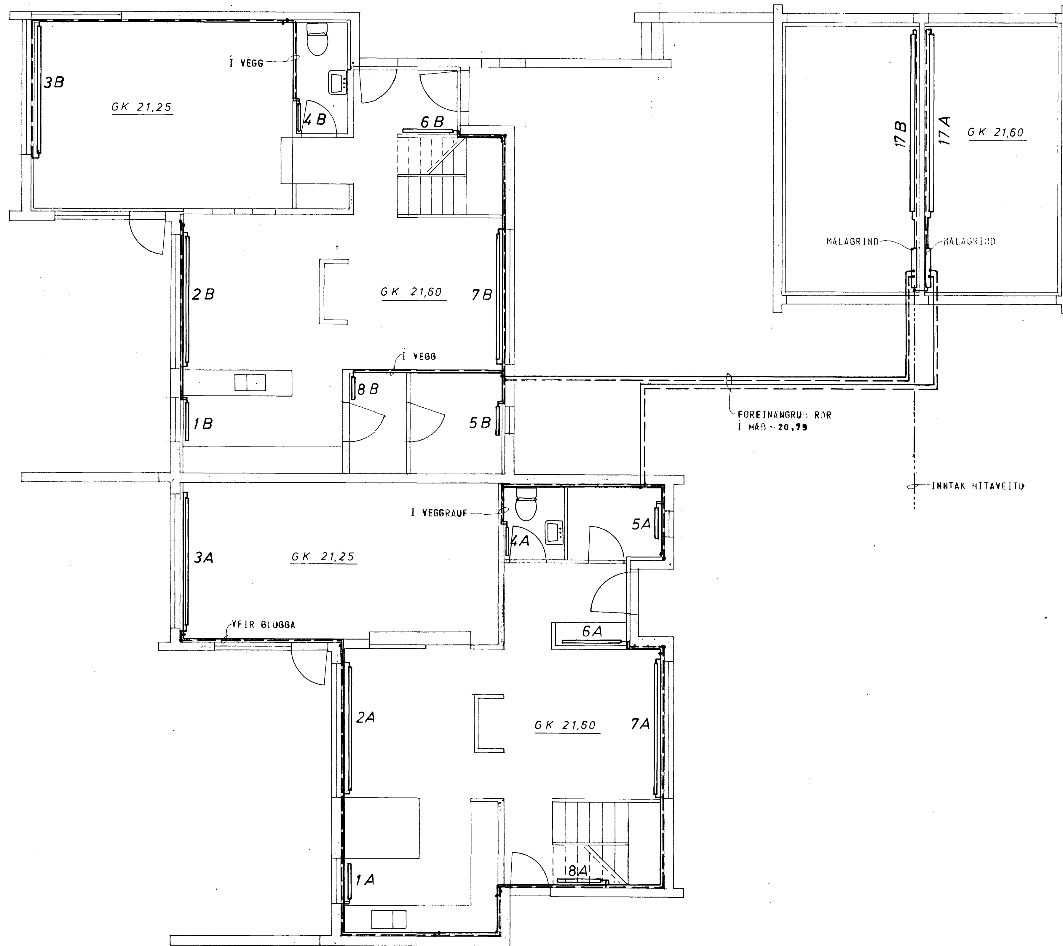
GRUNNMYND 1:50 1. HÆÐ
