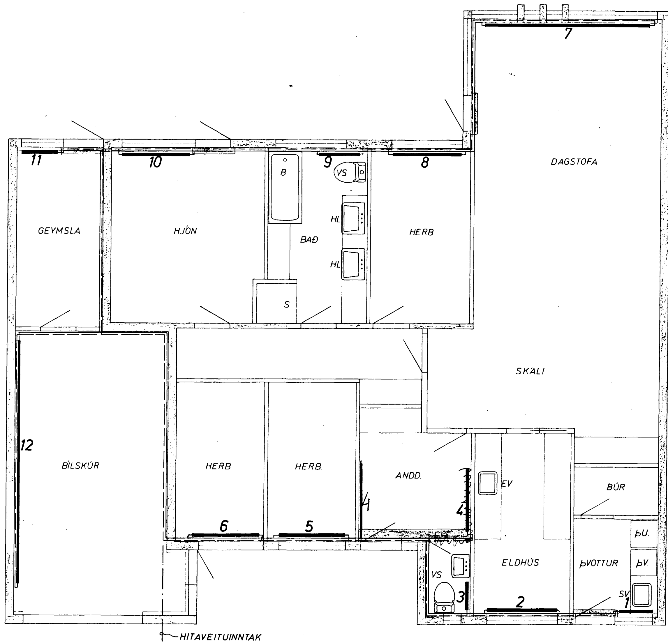
GRUNNMYND 1:50
