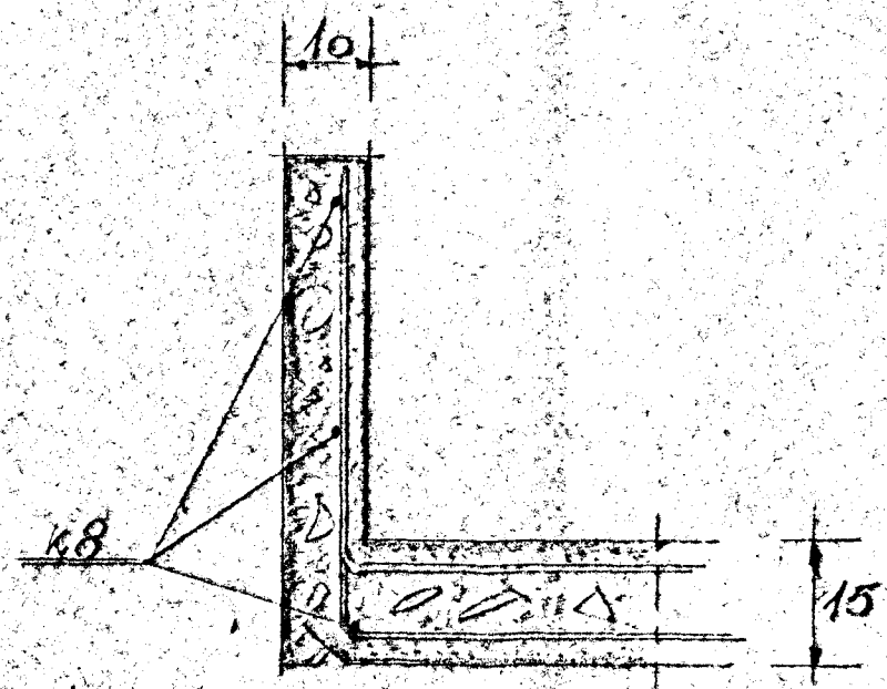
SNID A-A KVARN 1:10
