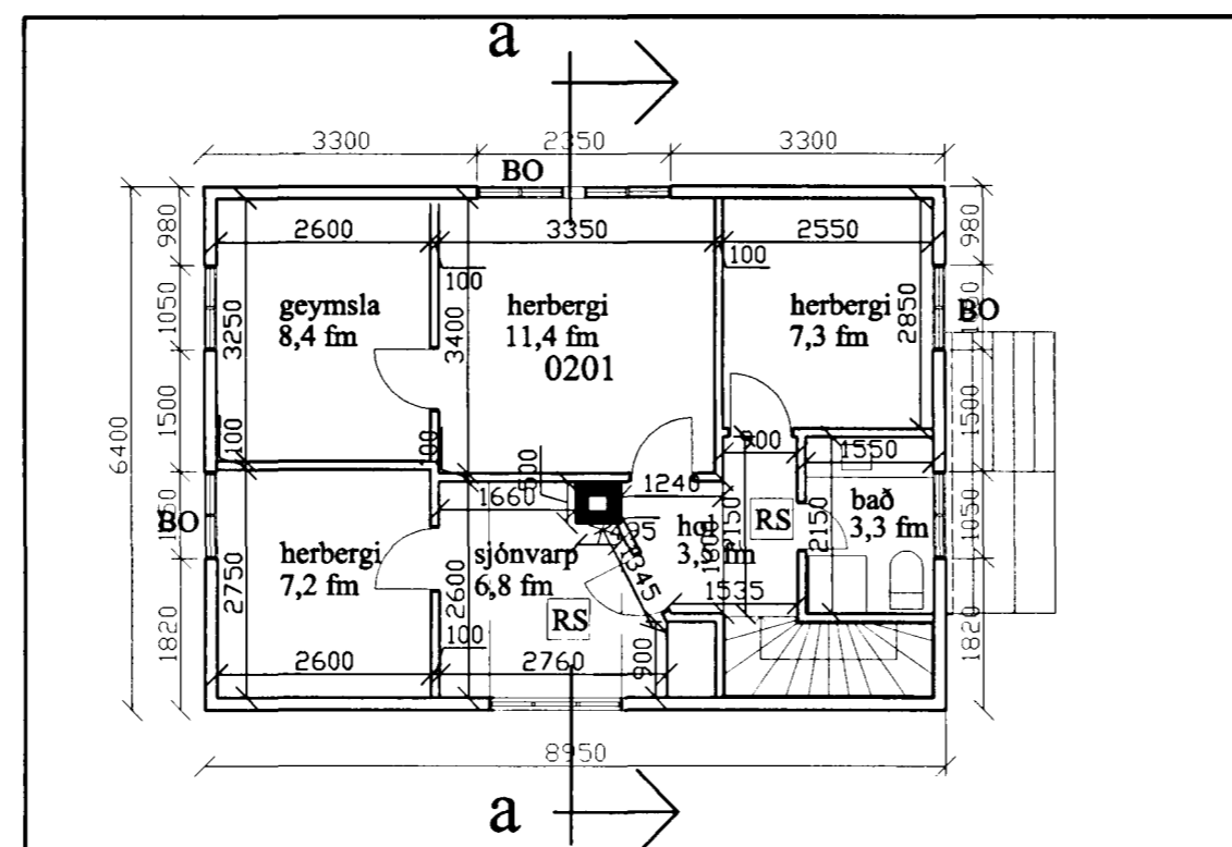
grunnmynd 2. hæð 1:100
