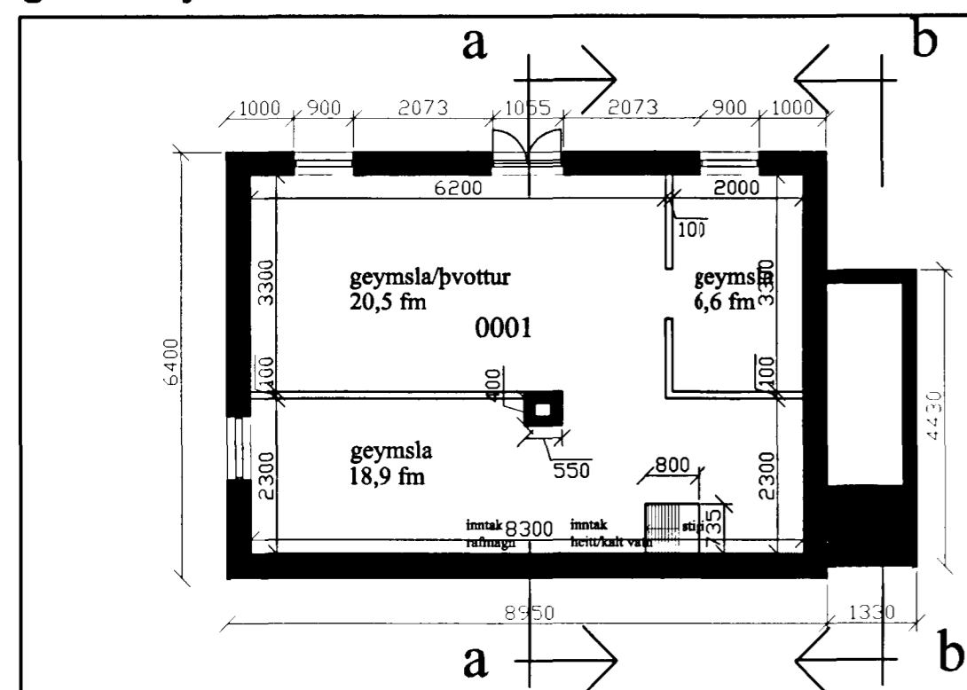
kjallari 1:100
