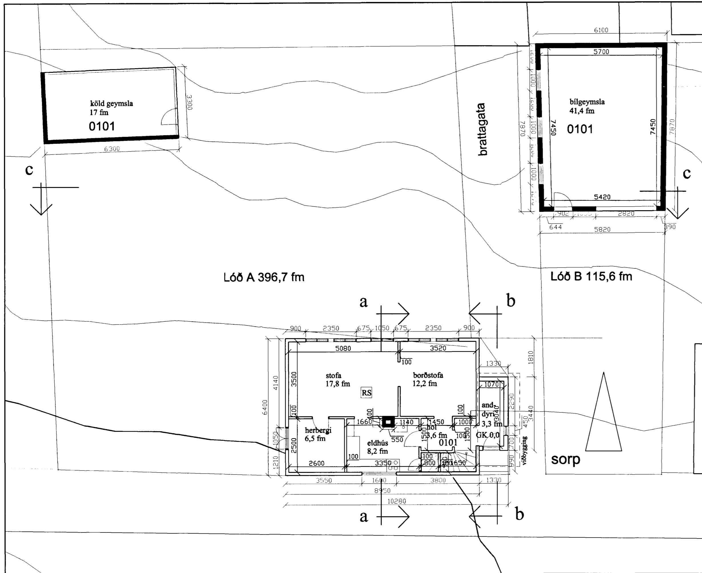
grunnmynd 1. hæð 1:100
