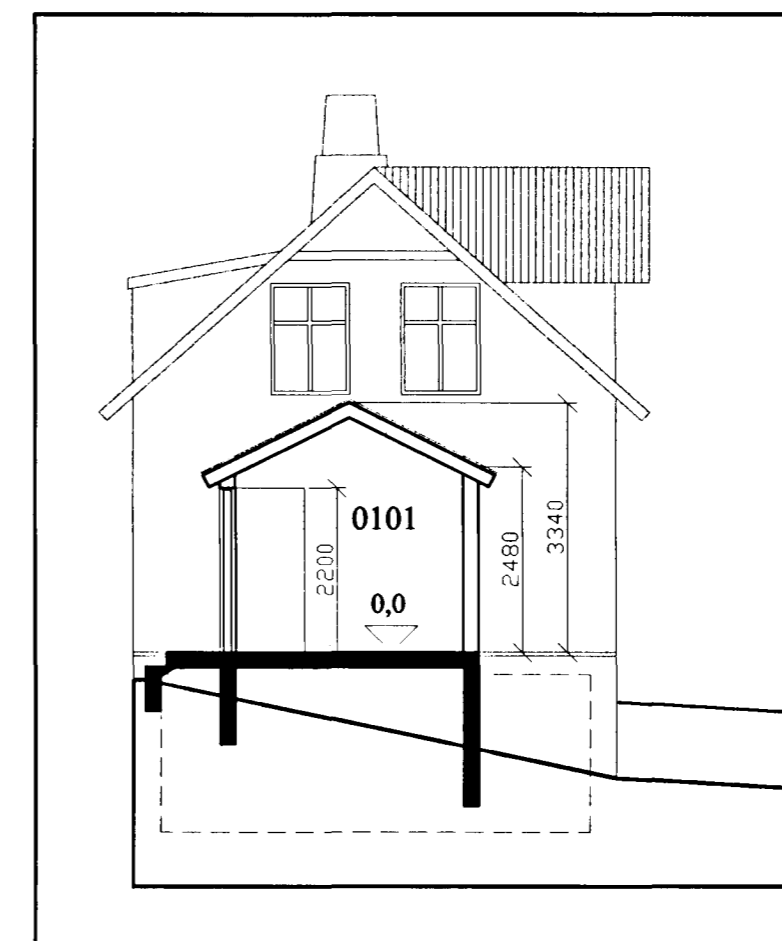
skurður b-b 1:100
