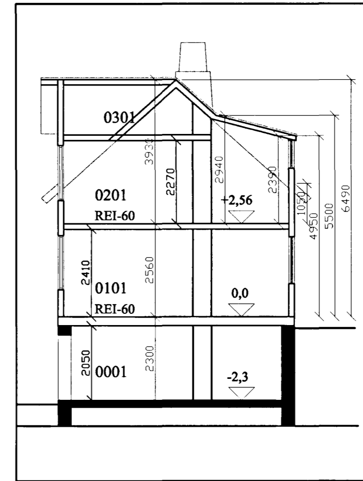
skurður a-a 1:100
