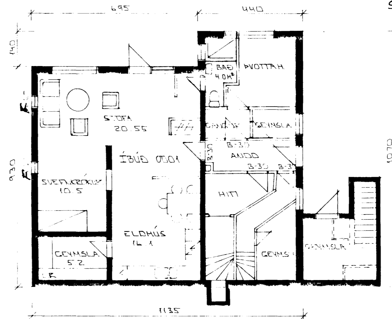
GRUNNMÝND KJALLARA
