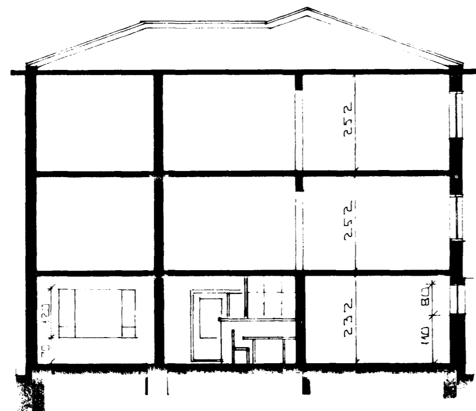
SNID • 1:100
