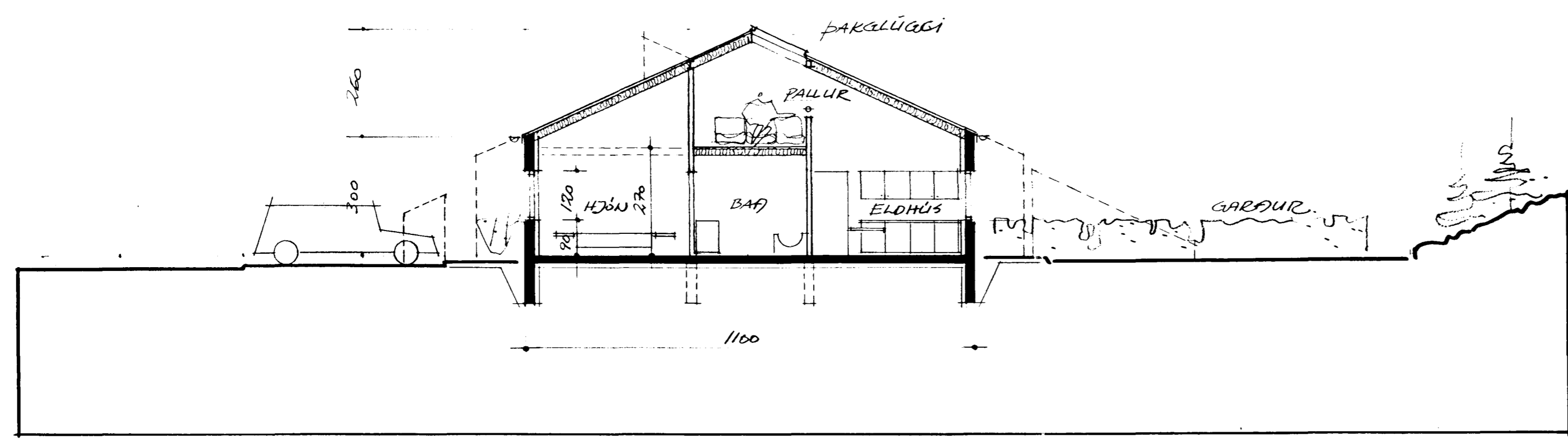
SKURÐUR A-A / 1:100
