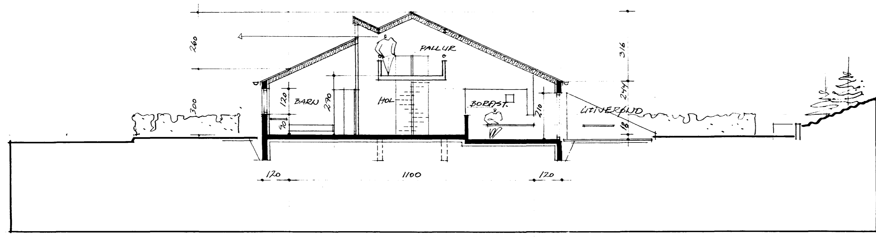
SKURÐUR B-B / 1:100
