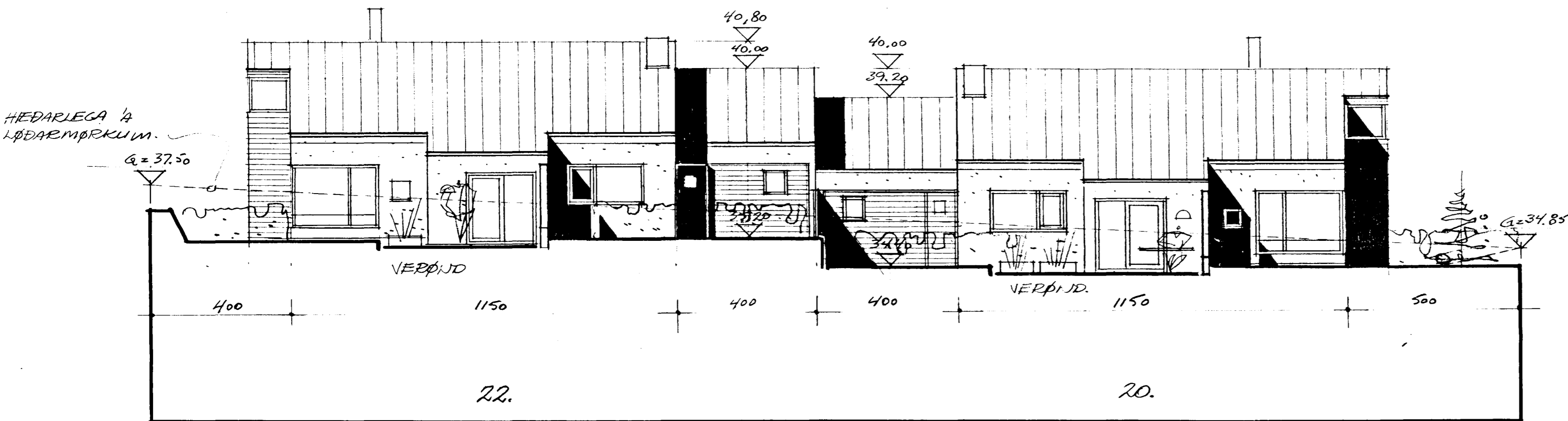
ÚTLIT SUÐUR 1:100
