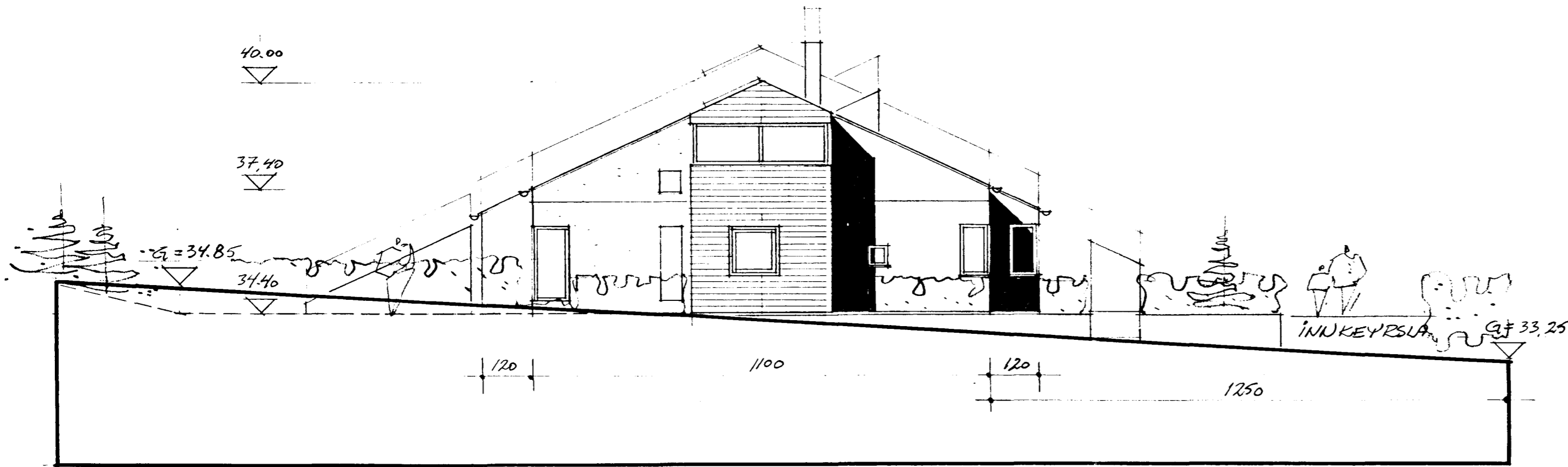
ÚTLIT AUSTUR 1:100
