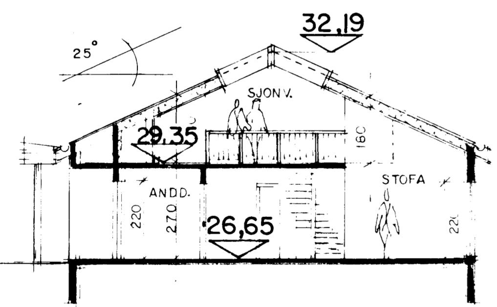
SKURÐUR A.A. 1:100
