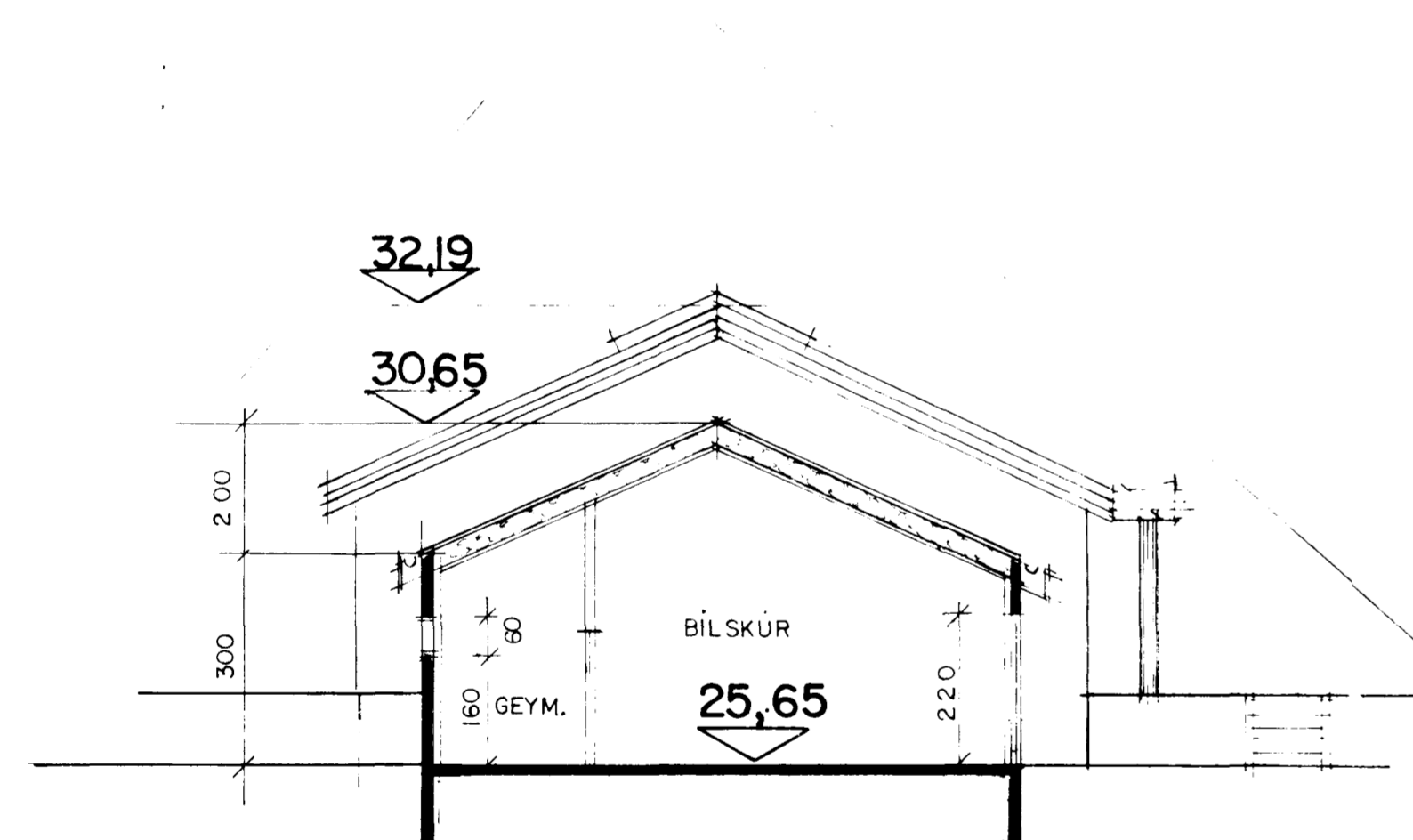
SKURÐUR B.B. 1:100
