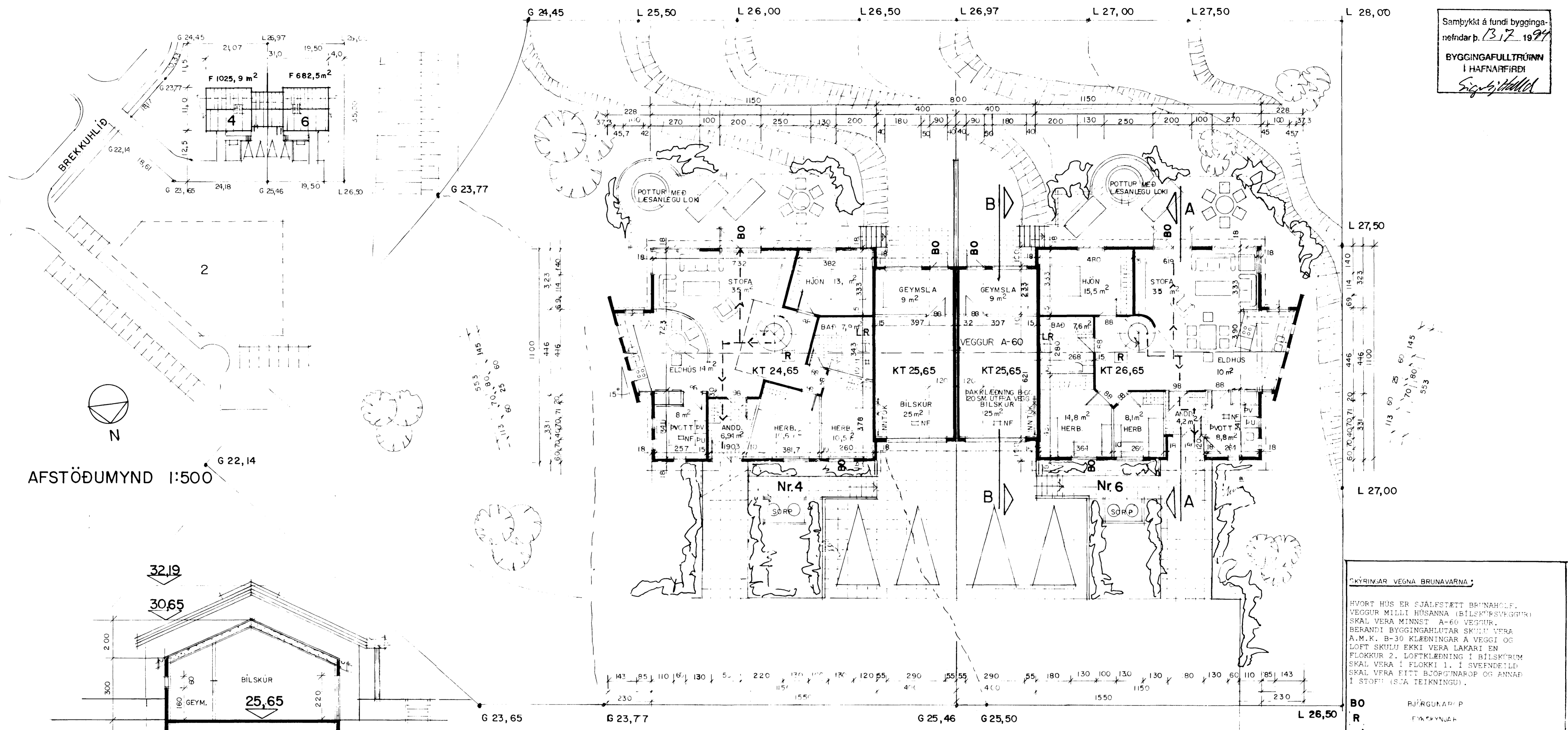
SKURÐUR B.B. 1:100
