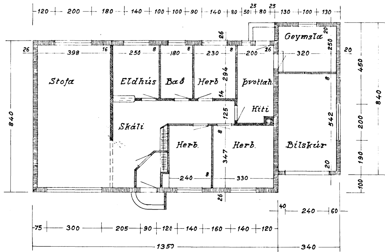
Grunnmynd.
