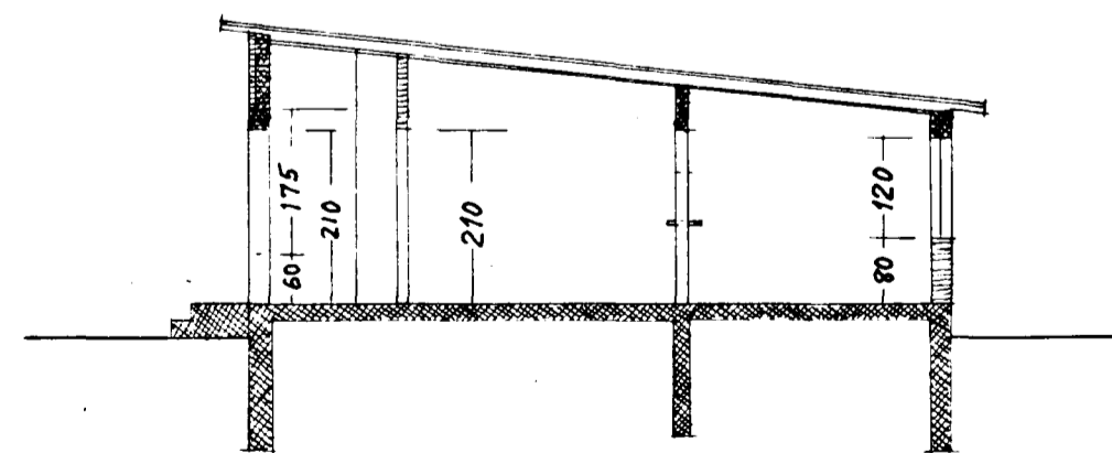
Þverskurður.
