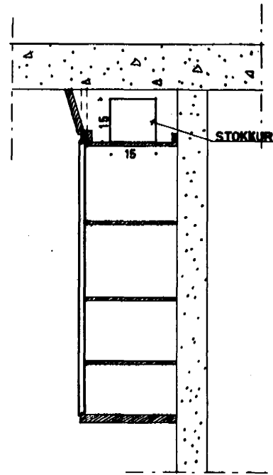
SNEIDING A-A
