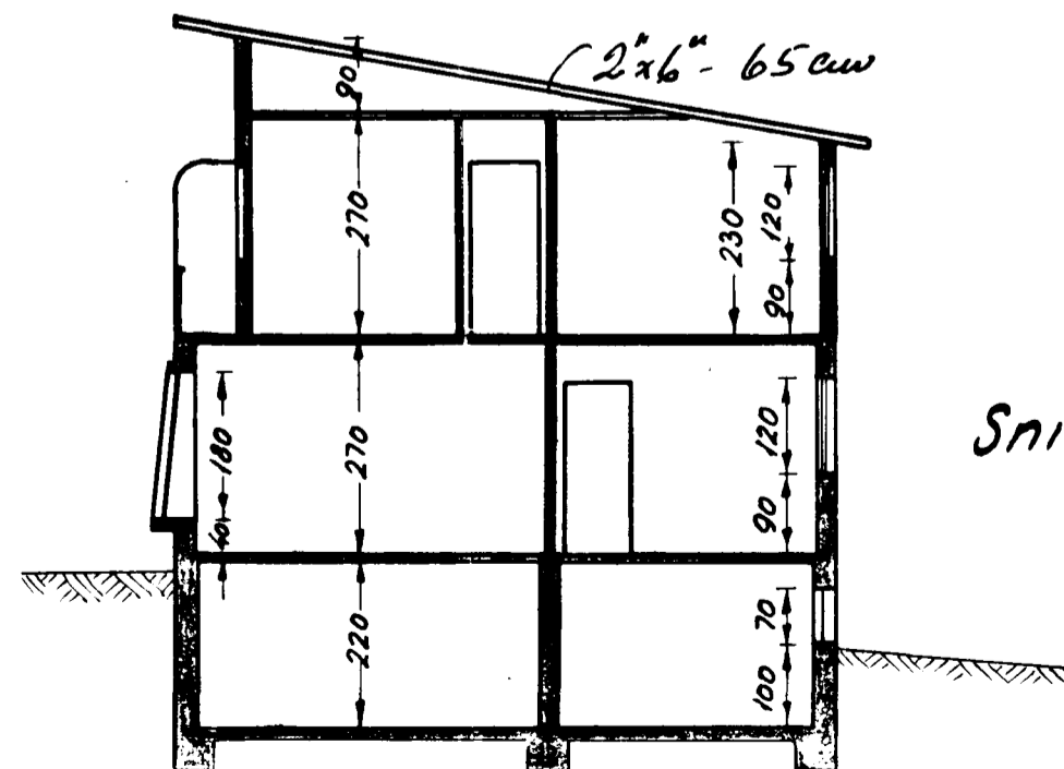
Bakhlíð
