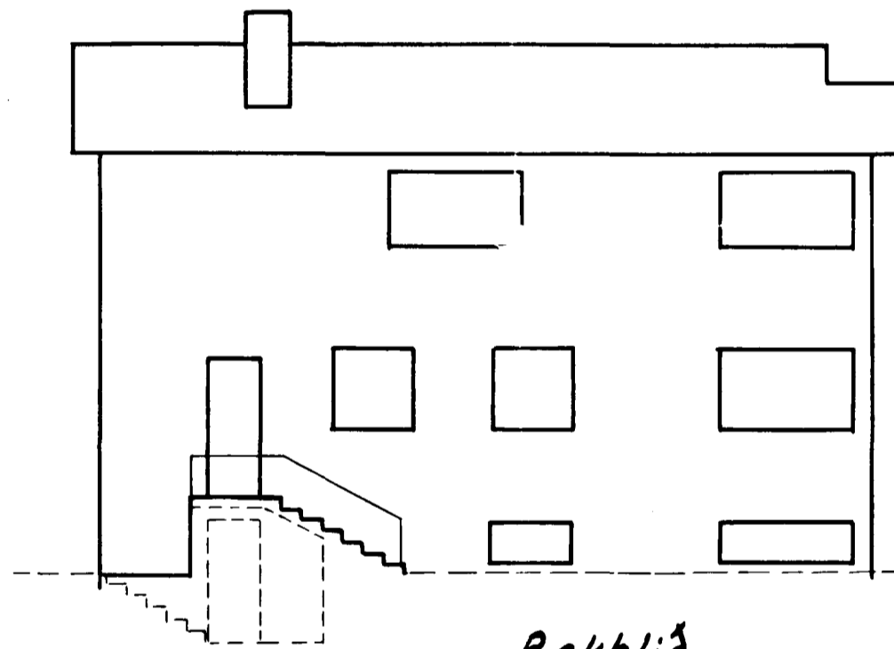
Bakhlíð
