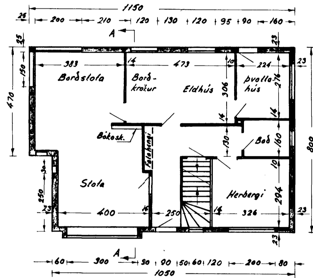
1. hæð
