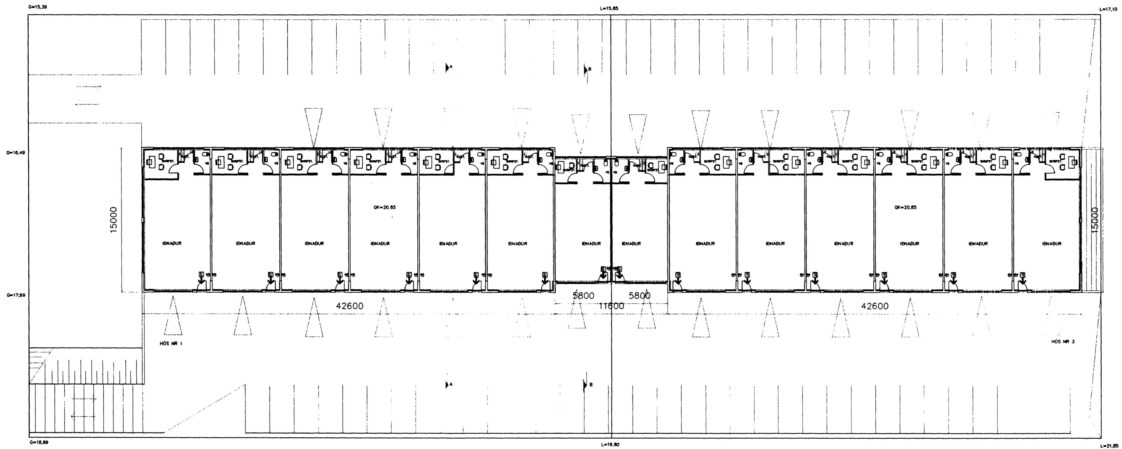
GRUNNMYND 2 HÆÐ.
