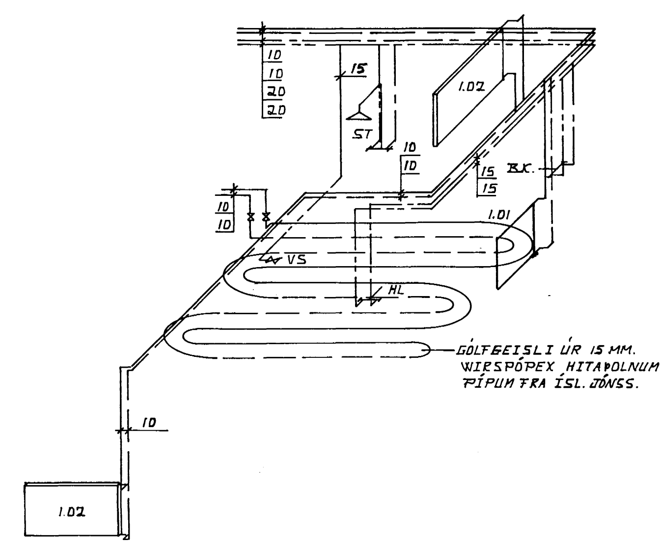
SNID Í GÖLFBEISLA. M. 1:10
