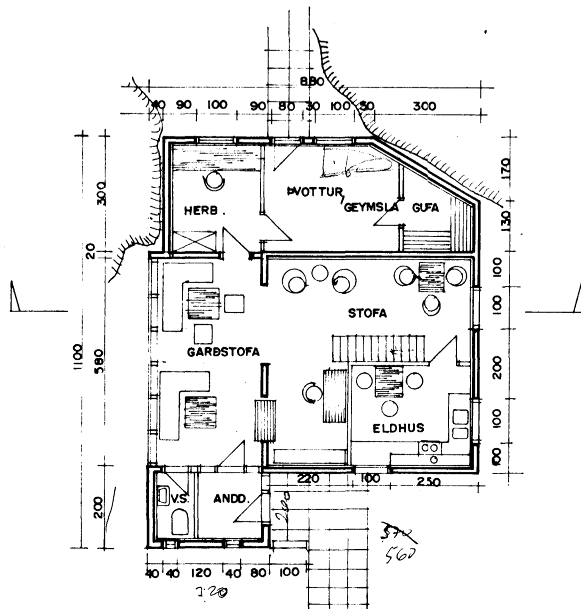
GRUNNMYND 1. HÆÐ M. 1:100
