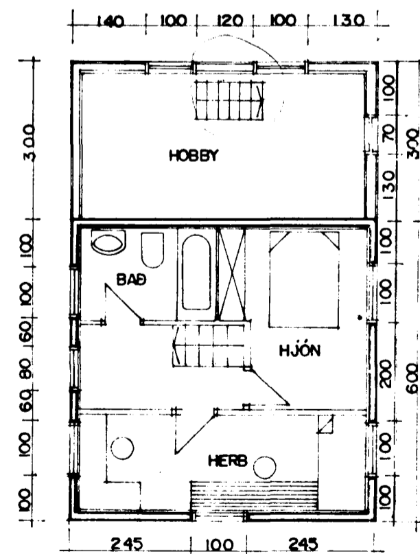
GRUNNMYND 2. HÆÐ M. 1:100
