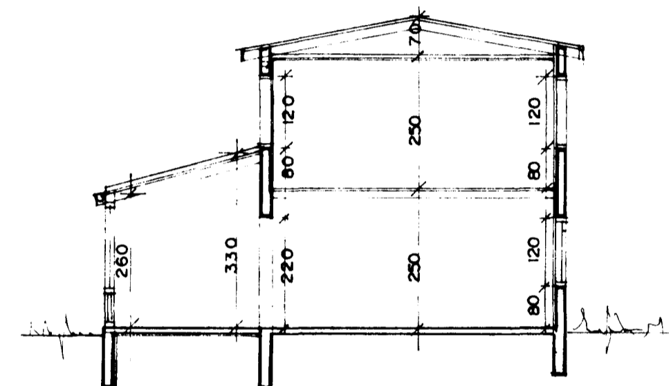
SNÍÐ A-A M. 1:100
