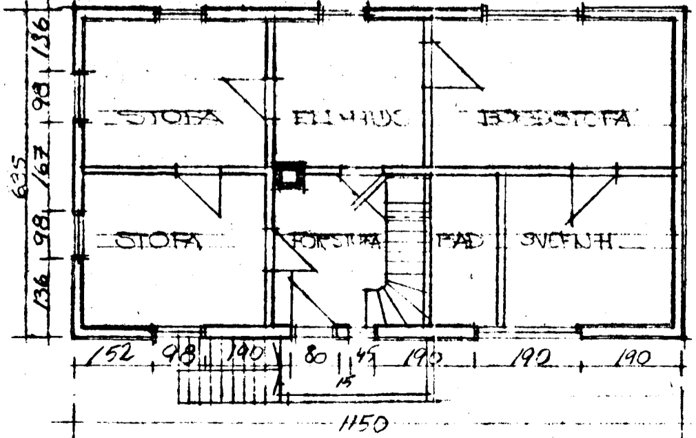
GEÖÐUMYND I FÆÐ M. 1:100
