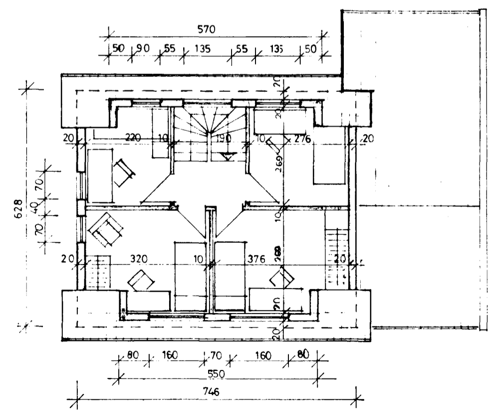
GRUNNMYND RISHÆÐAR 1:100
