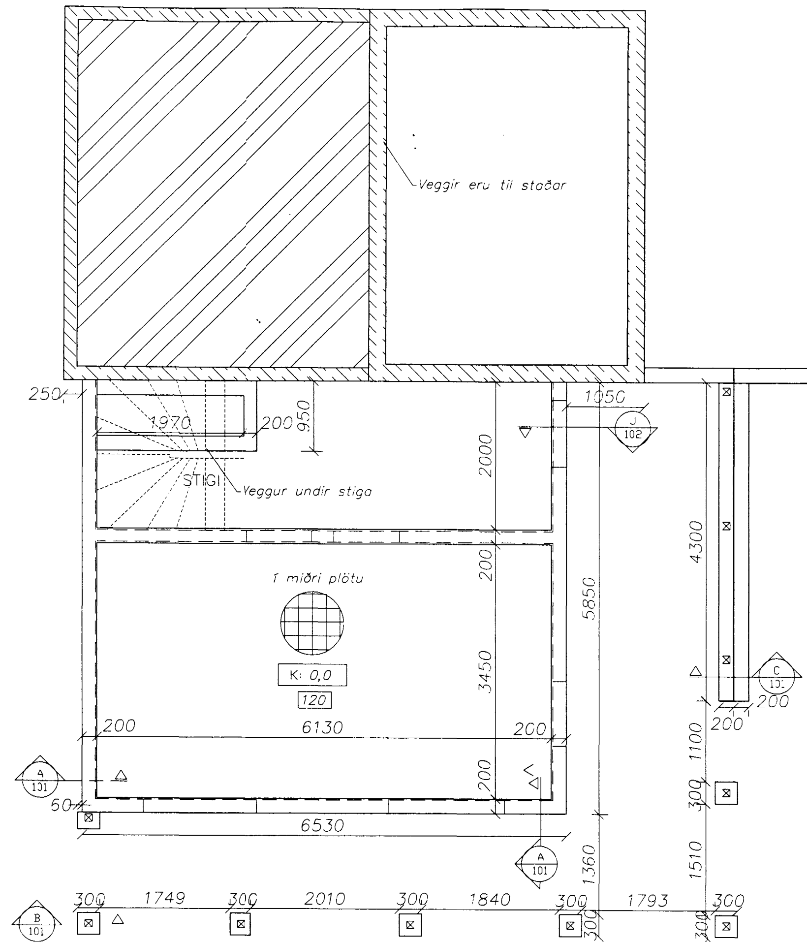
Grunnmynd Mælikvarði 1:50
