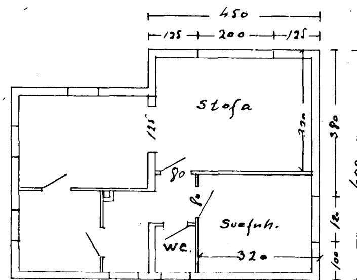
Grunnmynd.
