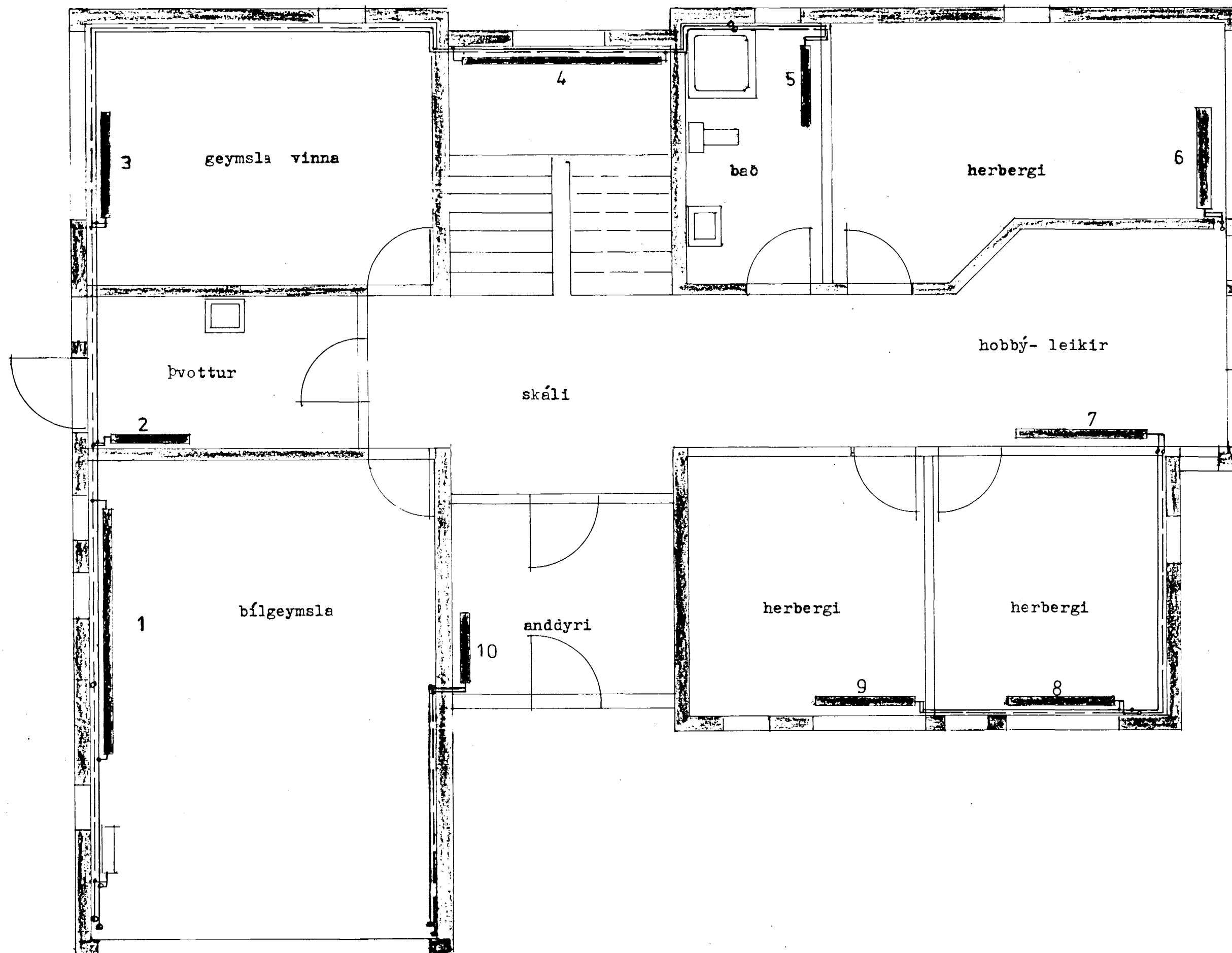
Hitakerfi grunnmynd neðri hæðar. M= 1:50
