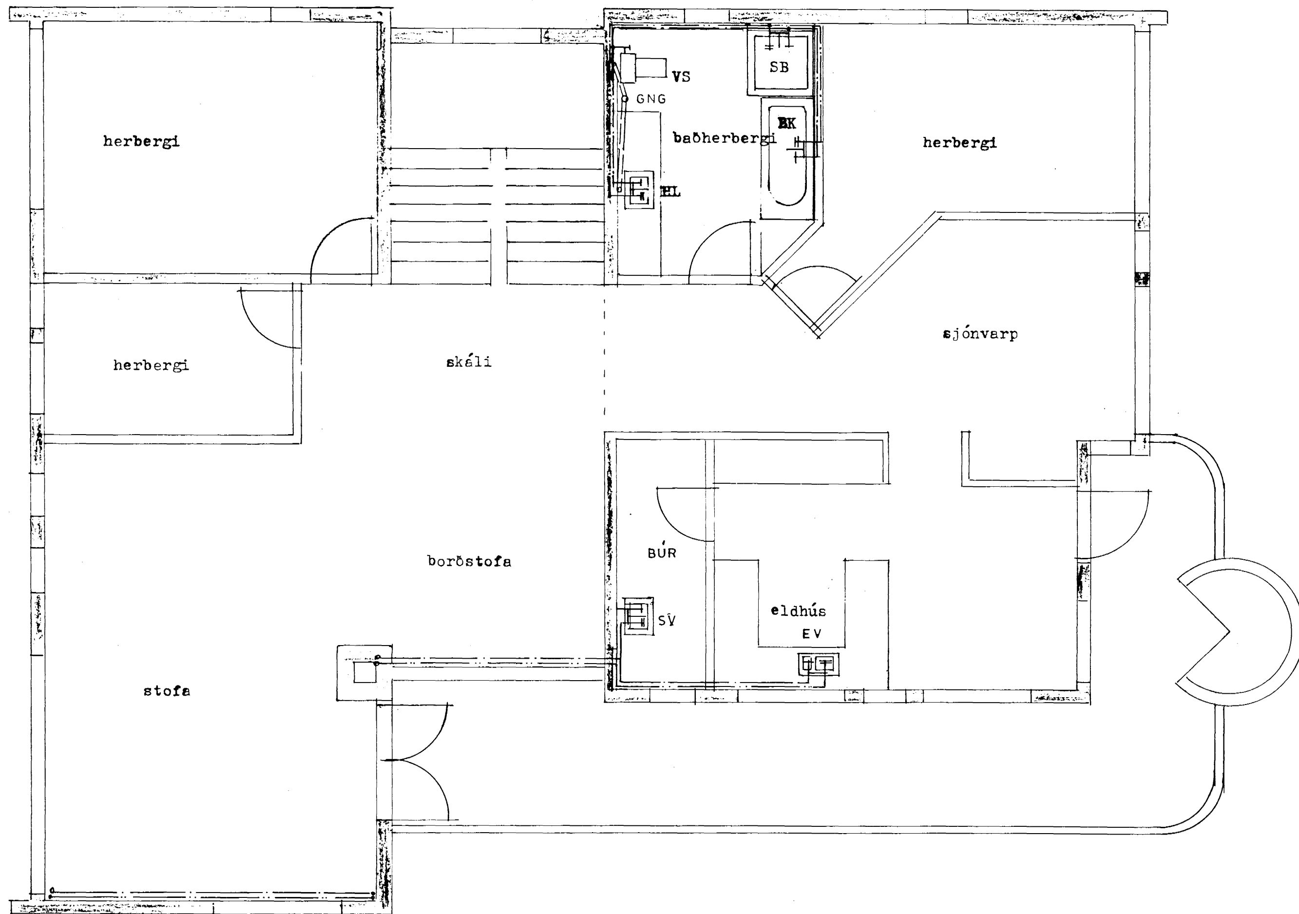
Neysluvatnskerfi, grunnmynd efri hæðar. M=1:50
