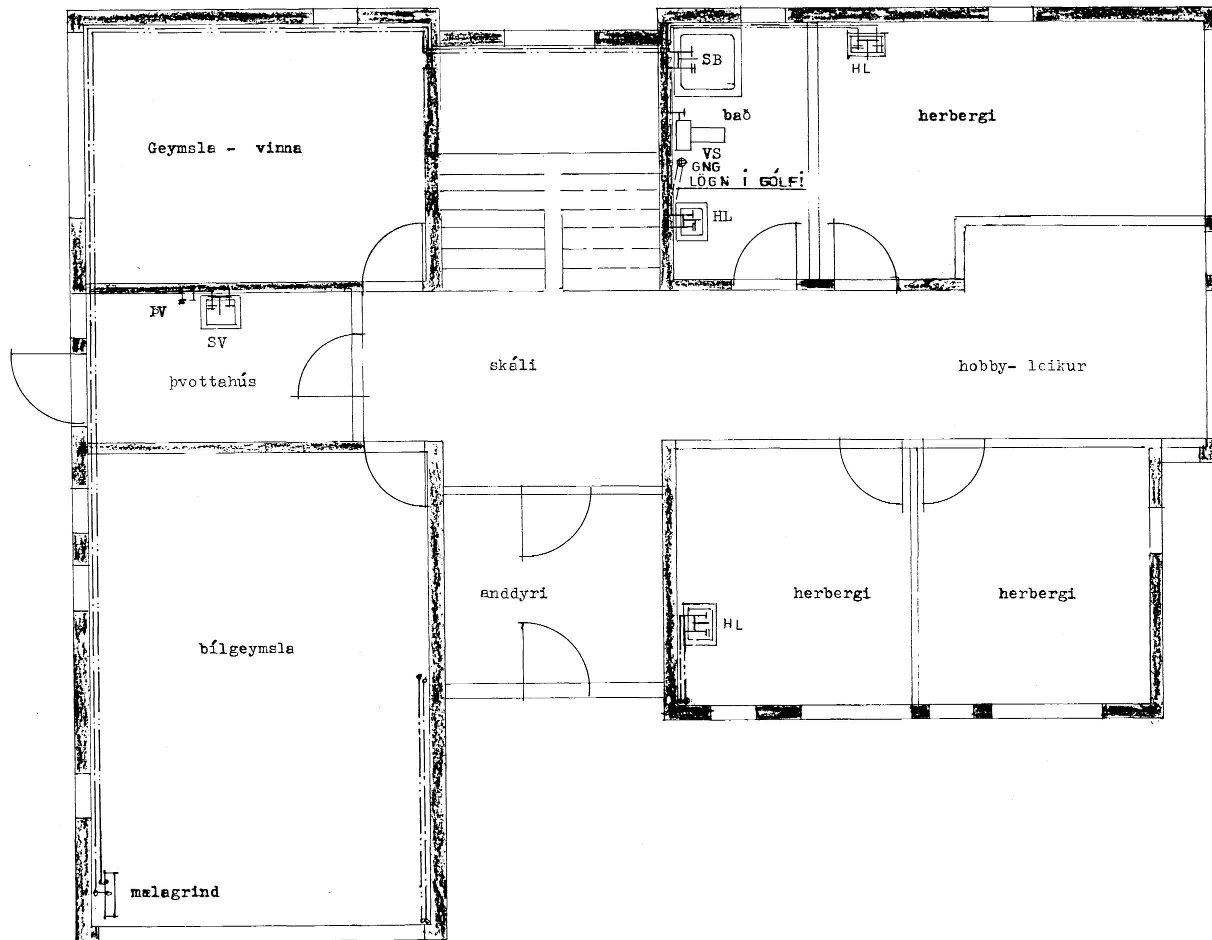
Neysluvatnslagnir neðri hæð, grunnmynd. M= 1:50
