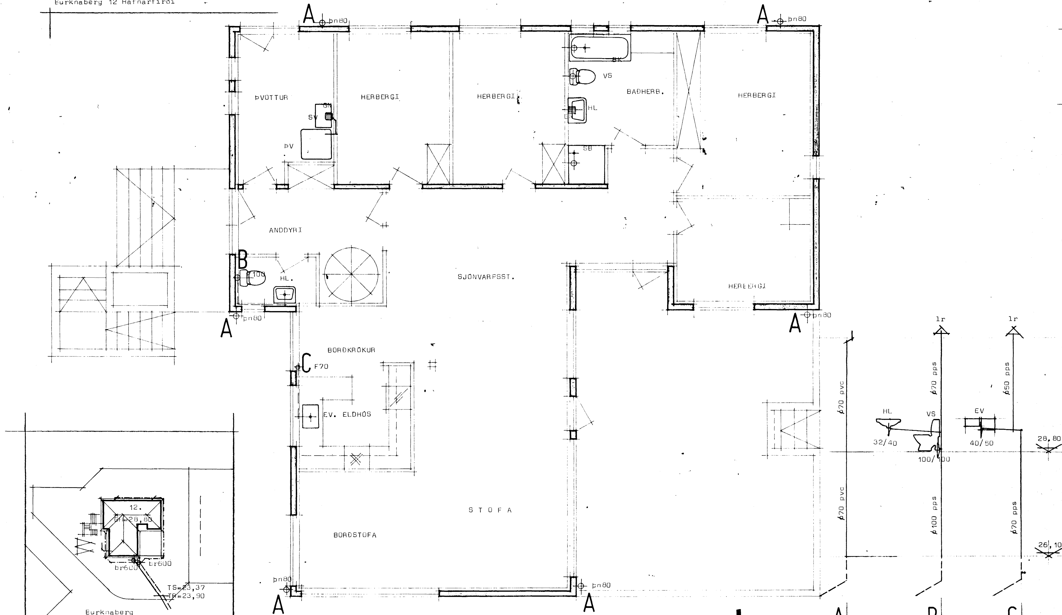
Grunnmynd hæðar Mk 1:50
