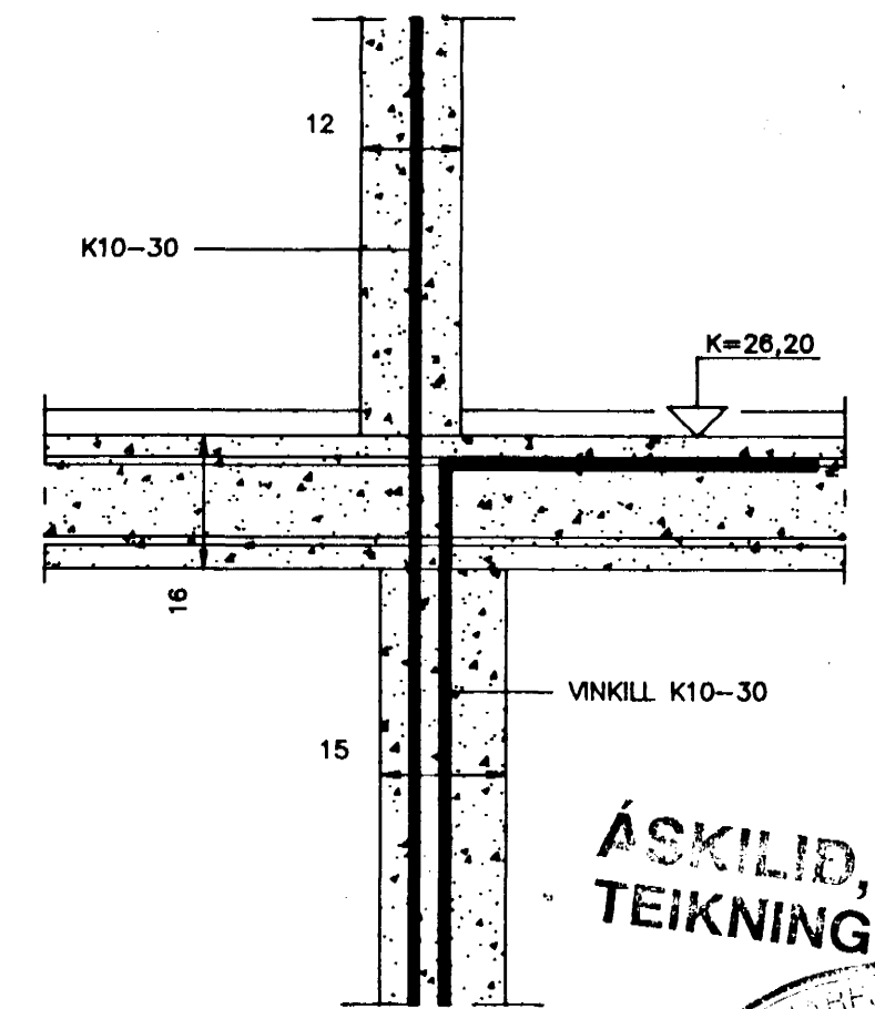
SNEIDING J
