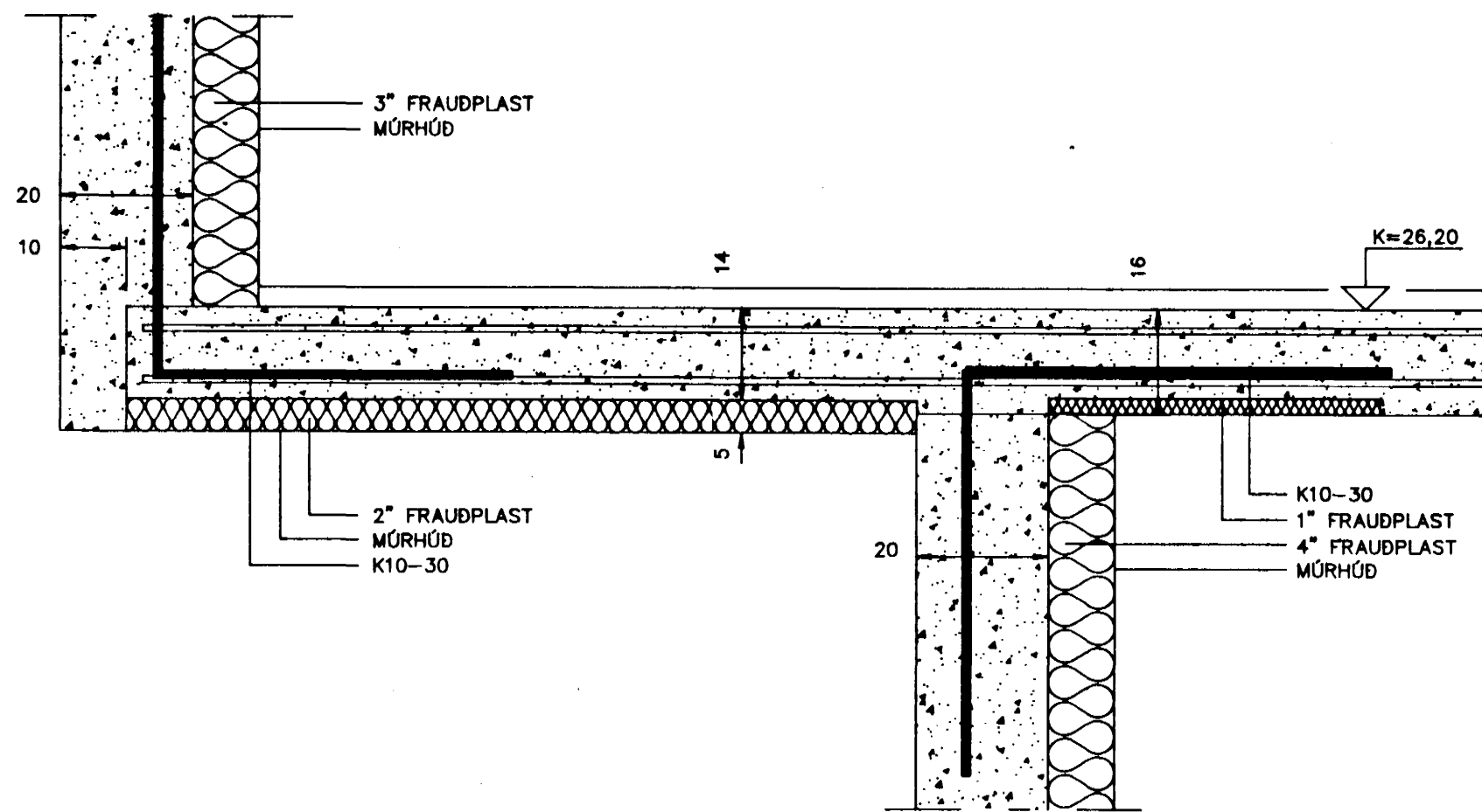
SNEIDING F
