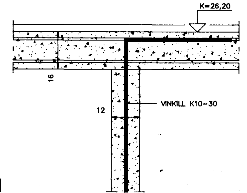
SNEIDING I
