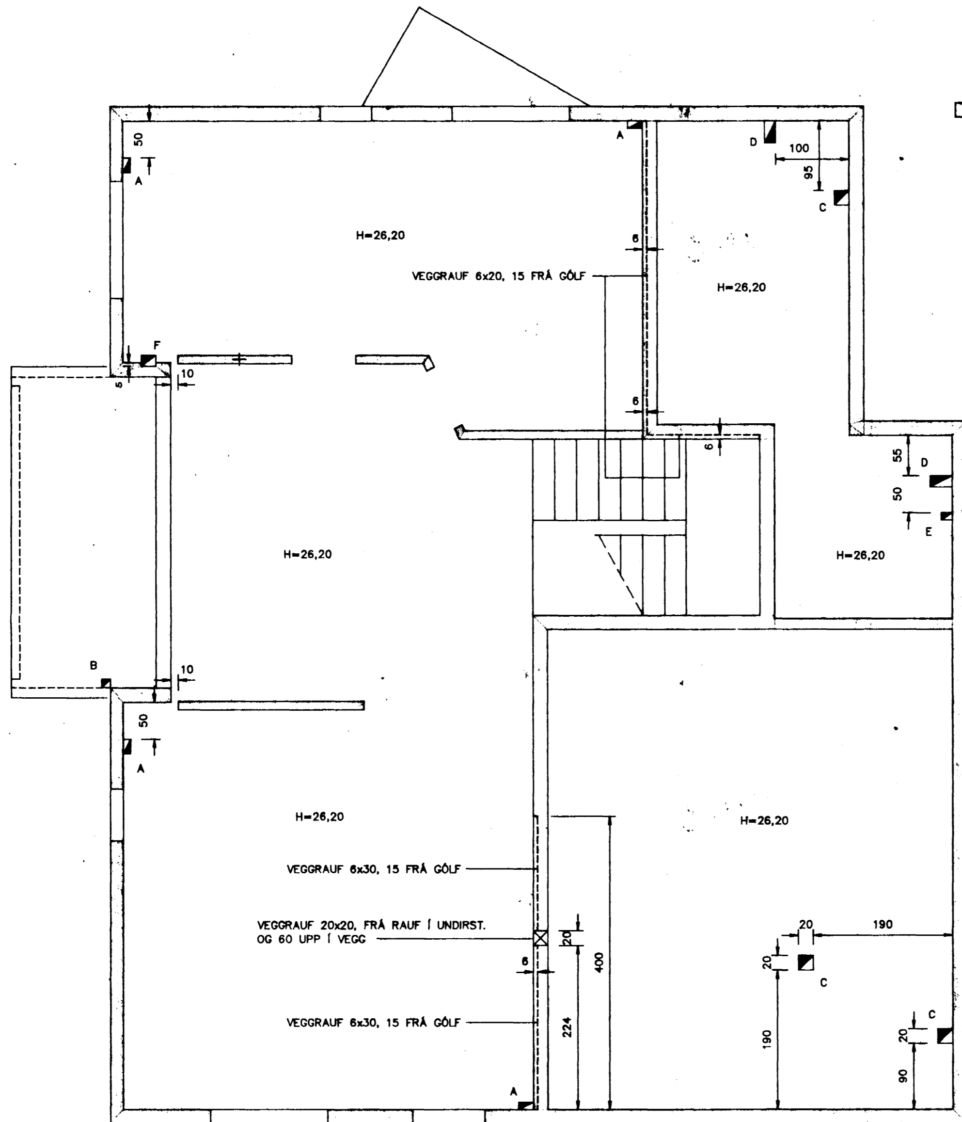
GRUNNMYND, M=1:50
