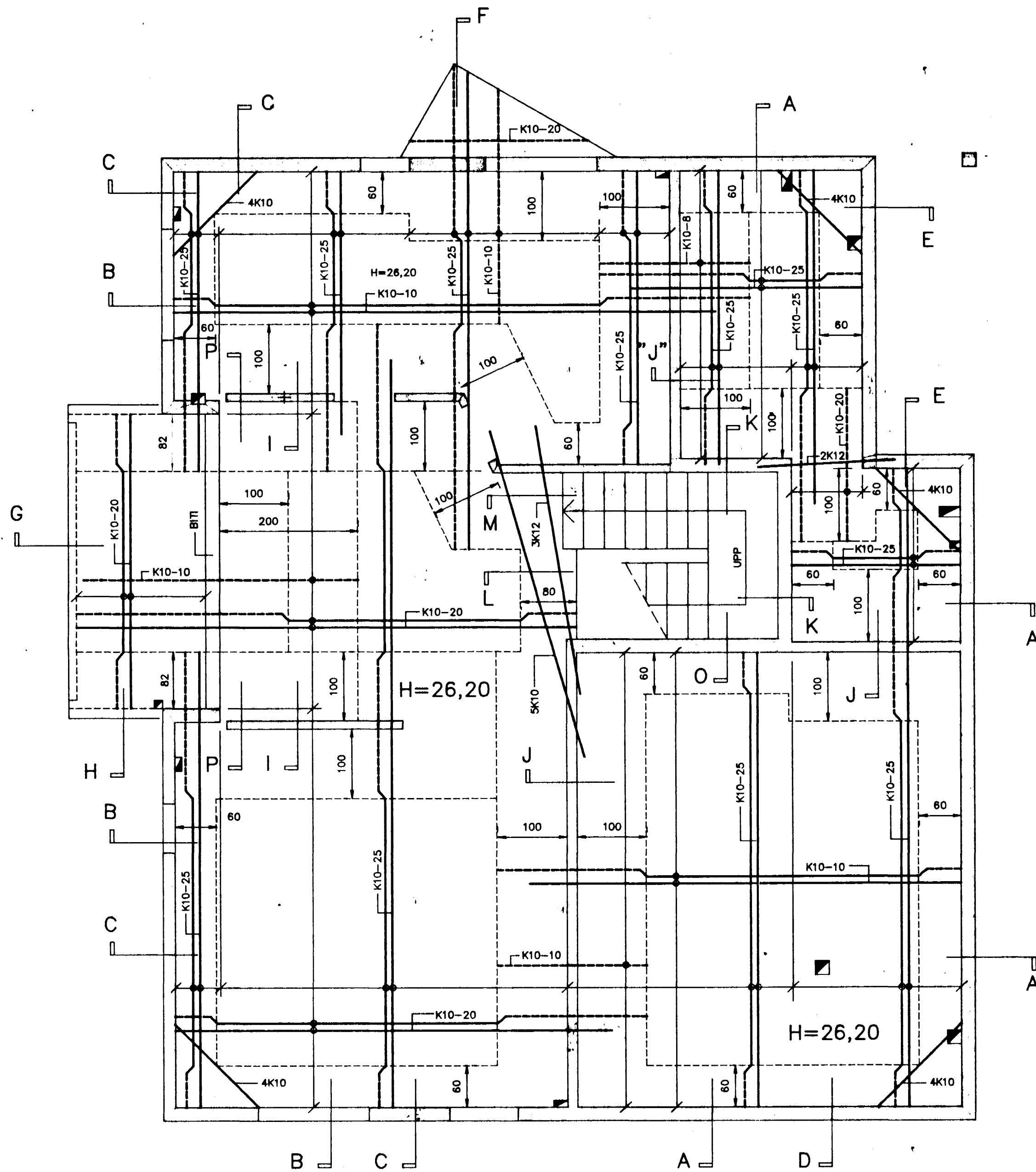
GRUNNMYND, M=1:50
