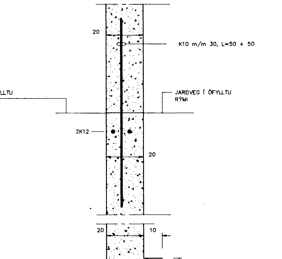
SNEIDING F
