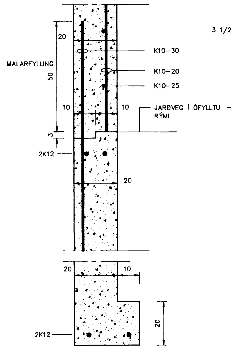
SNEIDING C
