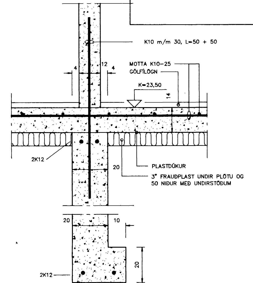
SNEIDING G
