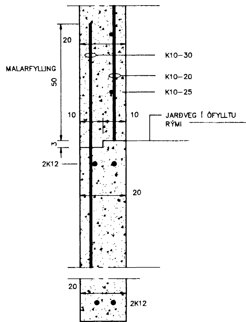
SNEIDING C
