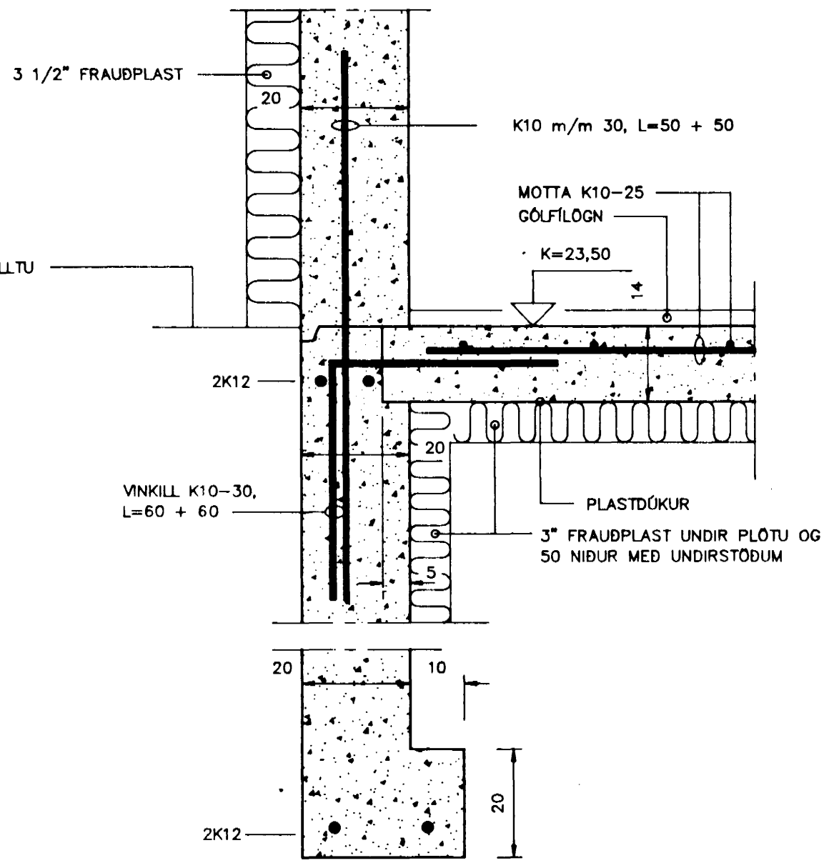
SNEIDING F
