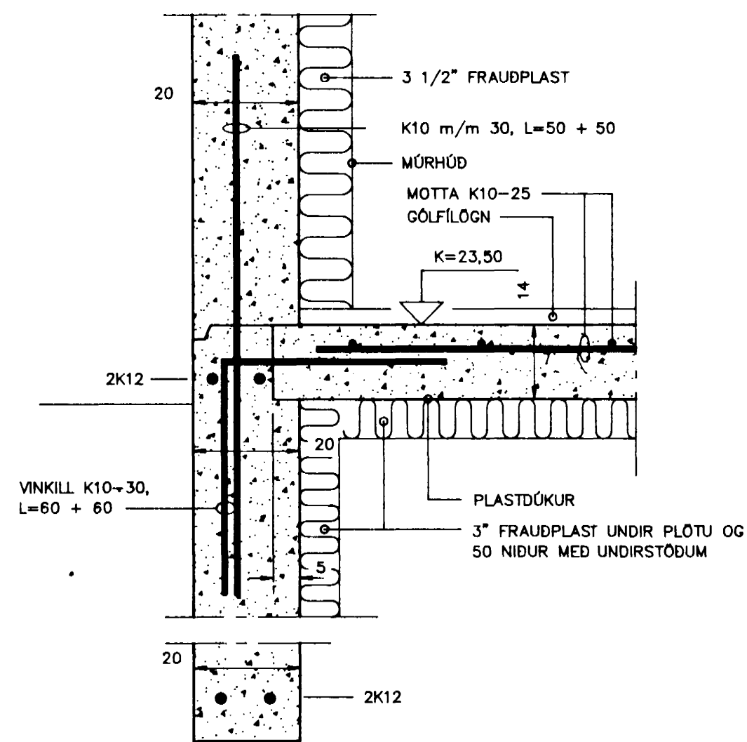
SNEIDING D
