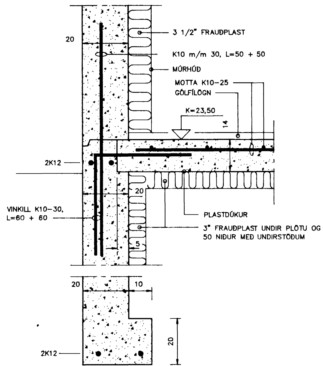
SNEIDING D
