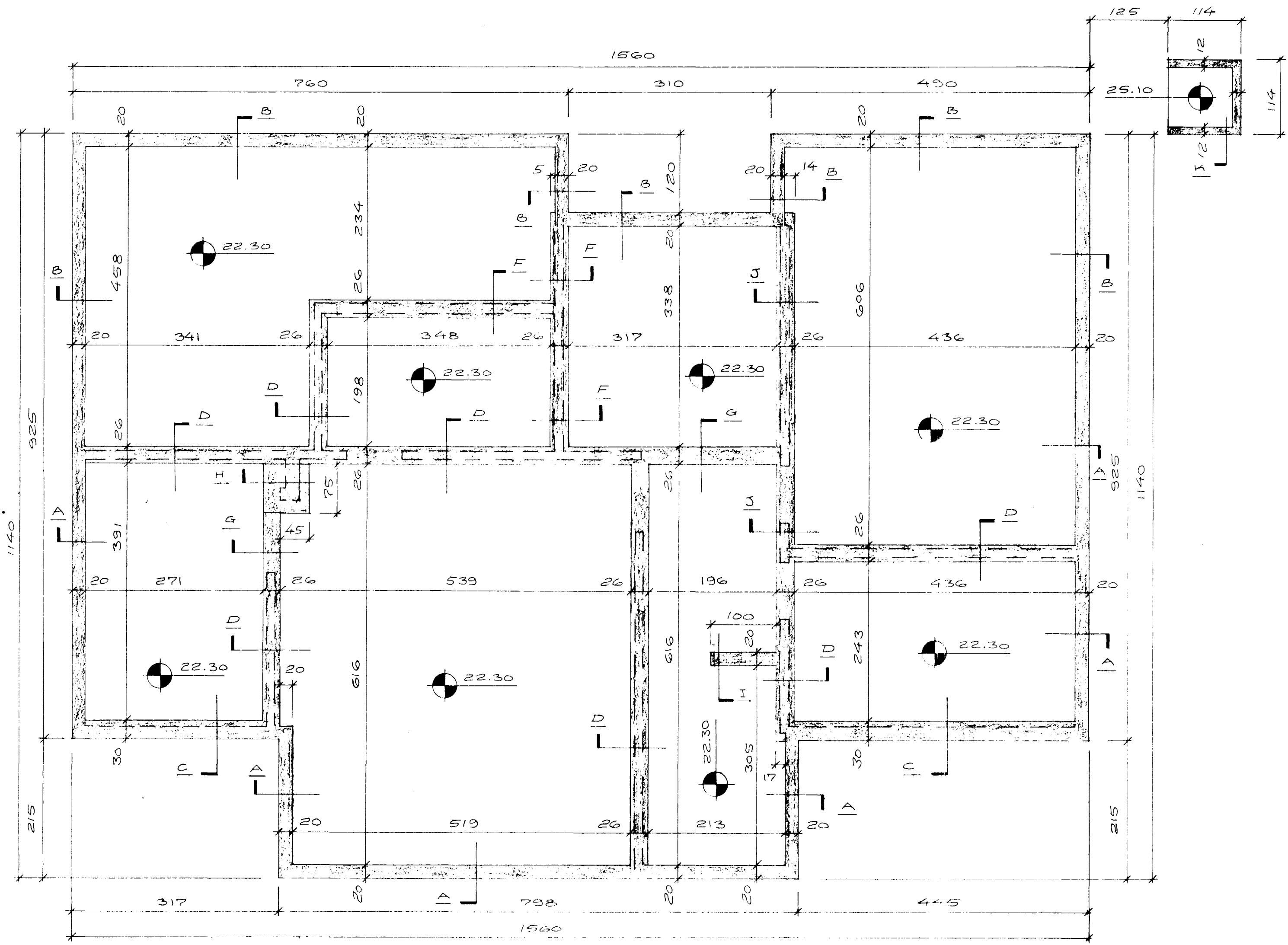
GRUNNMYND, M=1:50
