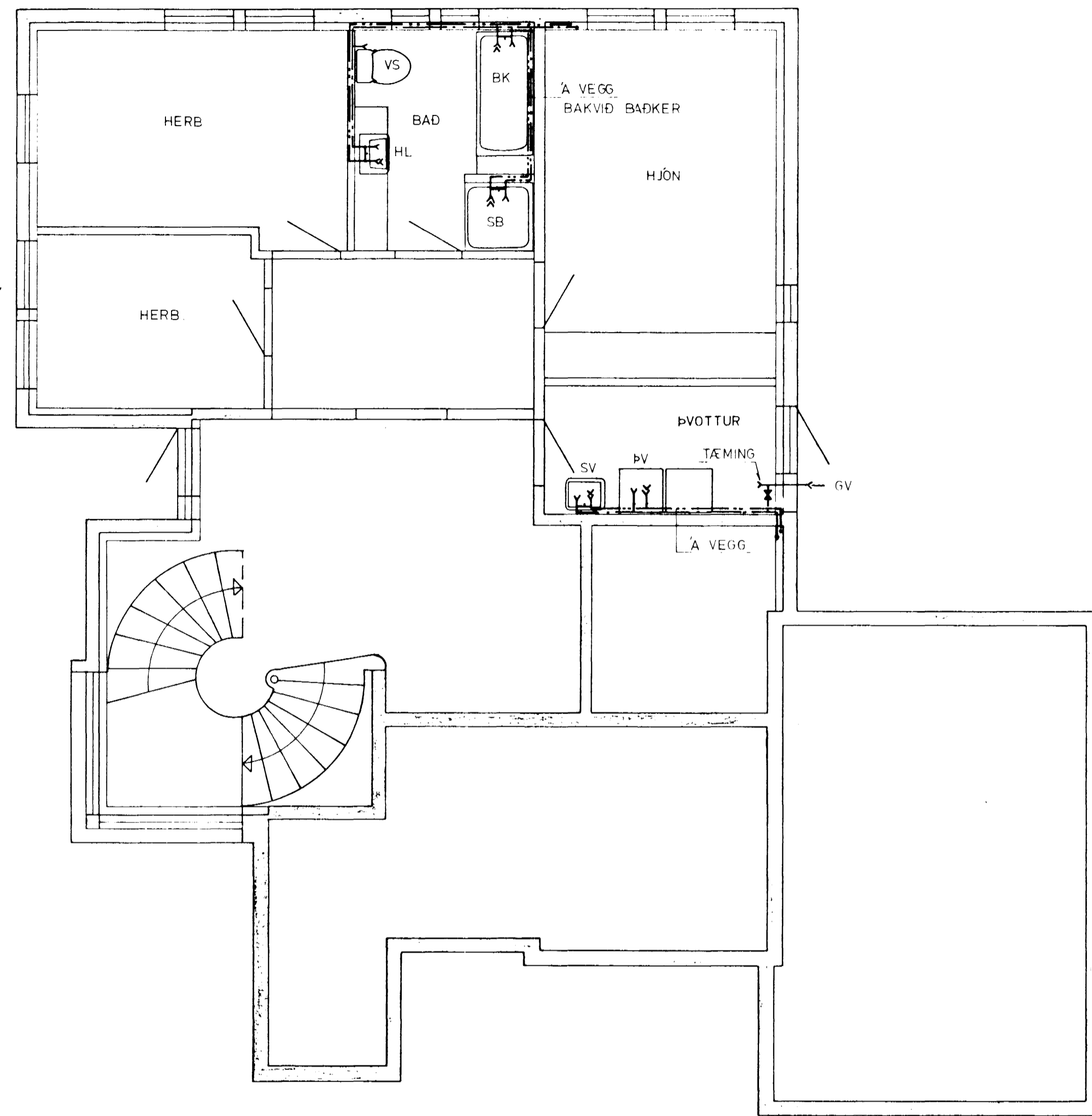
GRUNNMYND JARÐHÆÐAR 1:50
