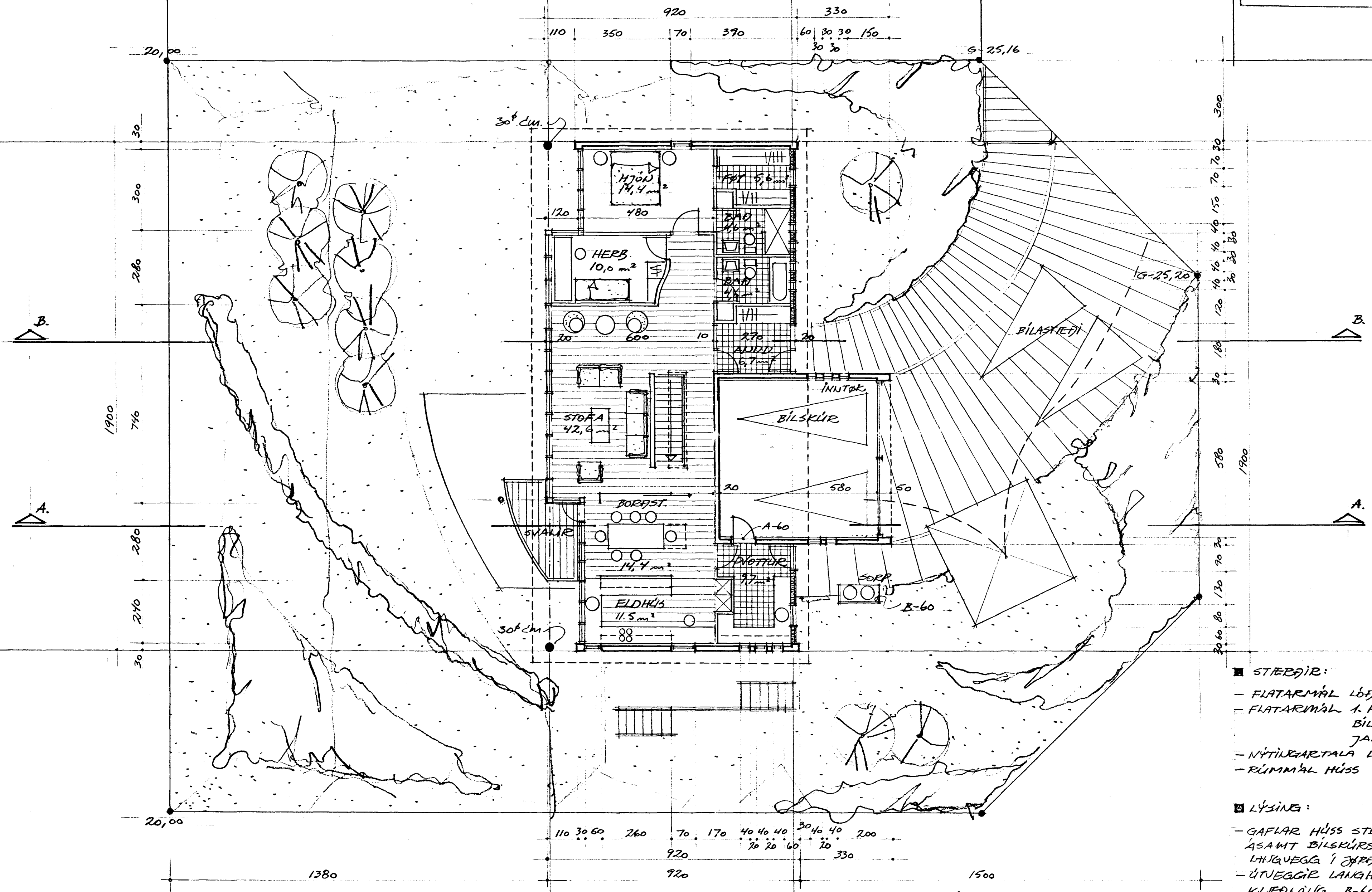
GRUNNMÝND 1. HÆÐ 1:100
