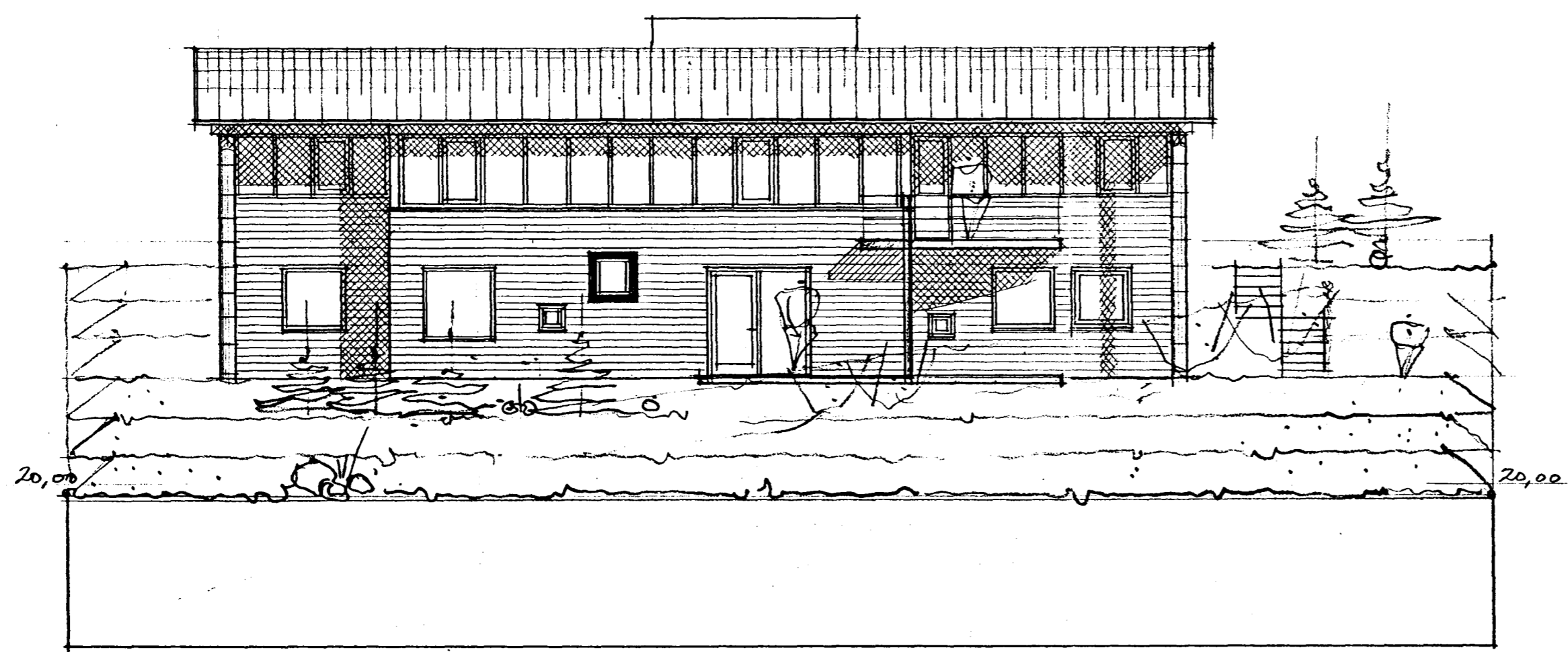
ÚTLIT SUÐUR.
