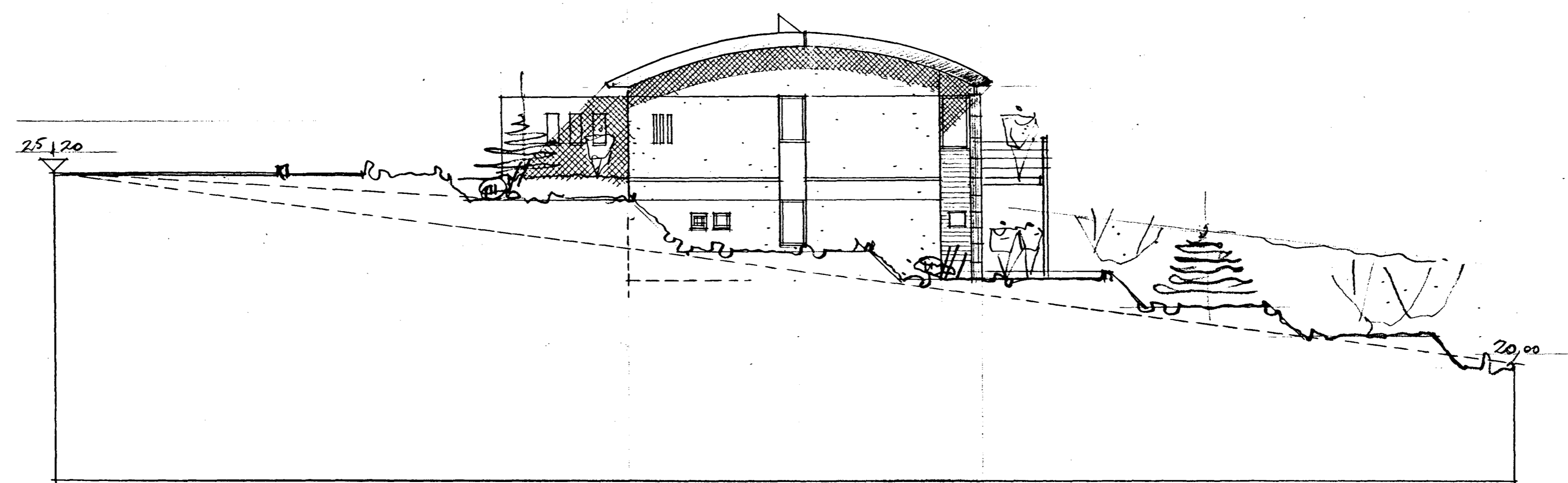
ÚTLIT VESTUR.
