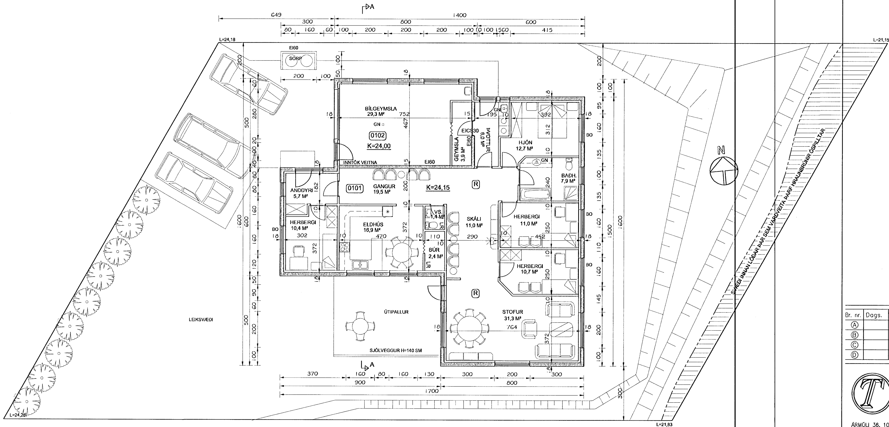
GRUNNMYND MKV. 1:100
