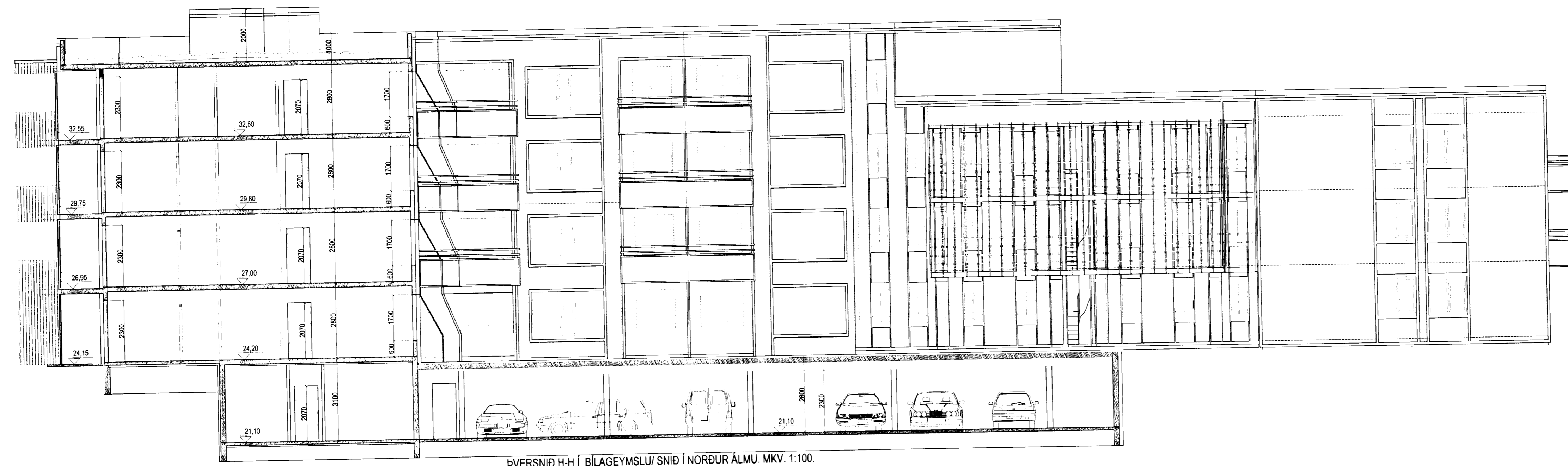
ÞVERSNID H-H Í BÍLAGEYMSLU/ SNID Í NORDUR ALMU. MKV. 1:100.
