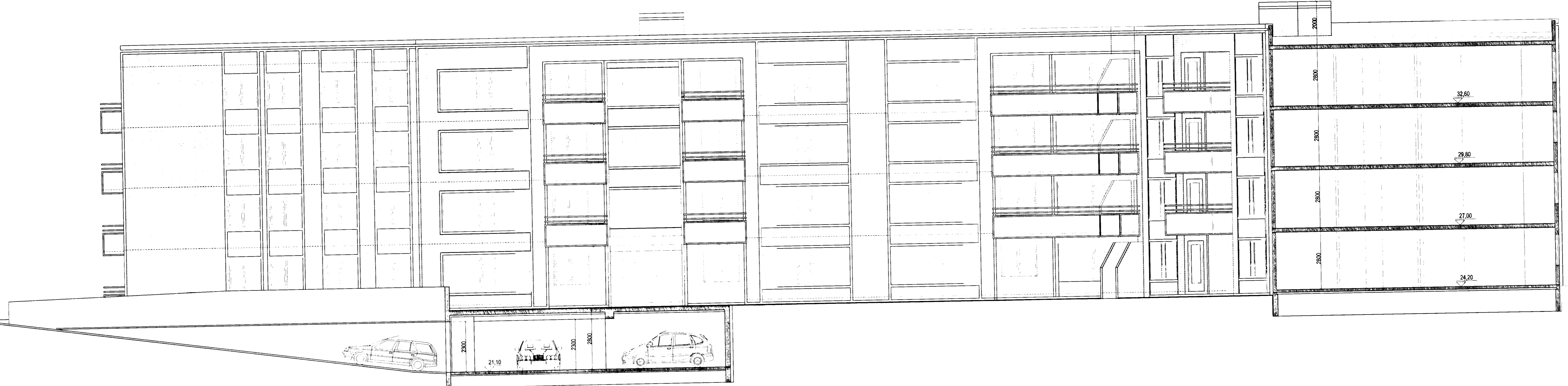
SNID F-F Í INNKEYRSLU BÍLAGEYMSLU. MKV. 1:100.
