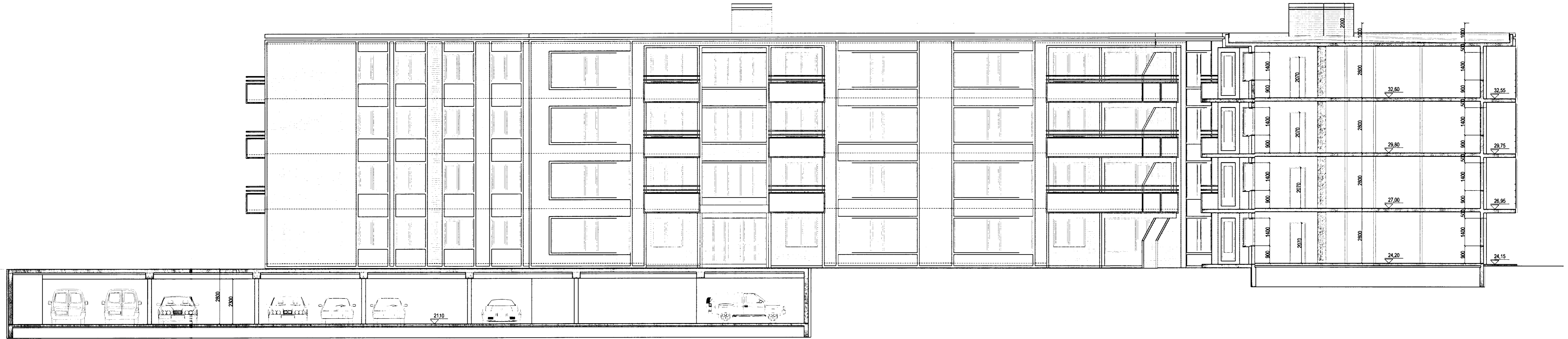
LANGSNÍÐ G-G Í BÍLAGEYMSLU. MKV. 1:100.
