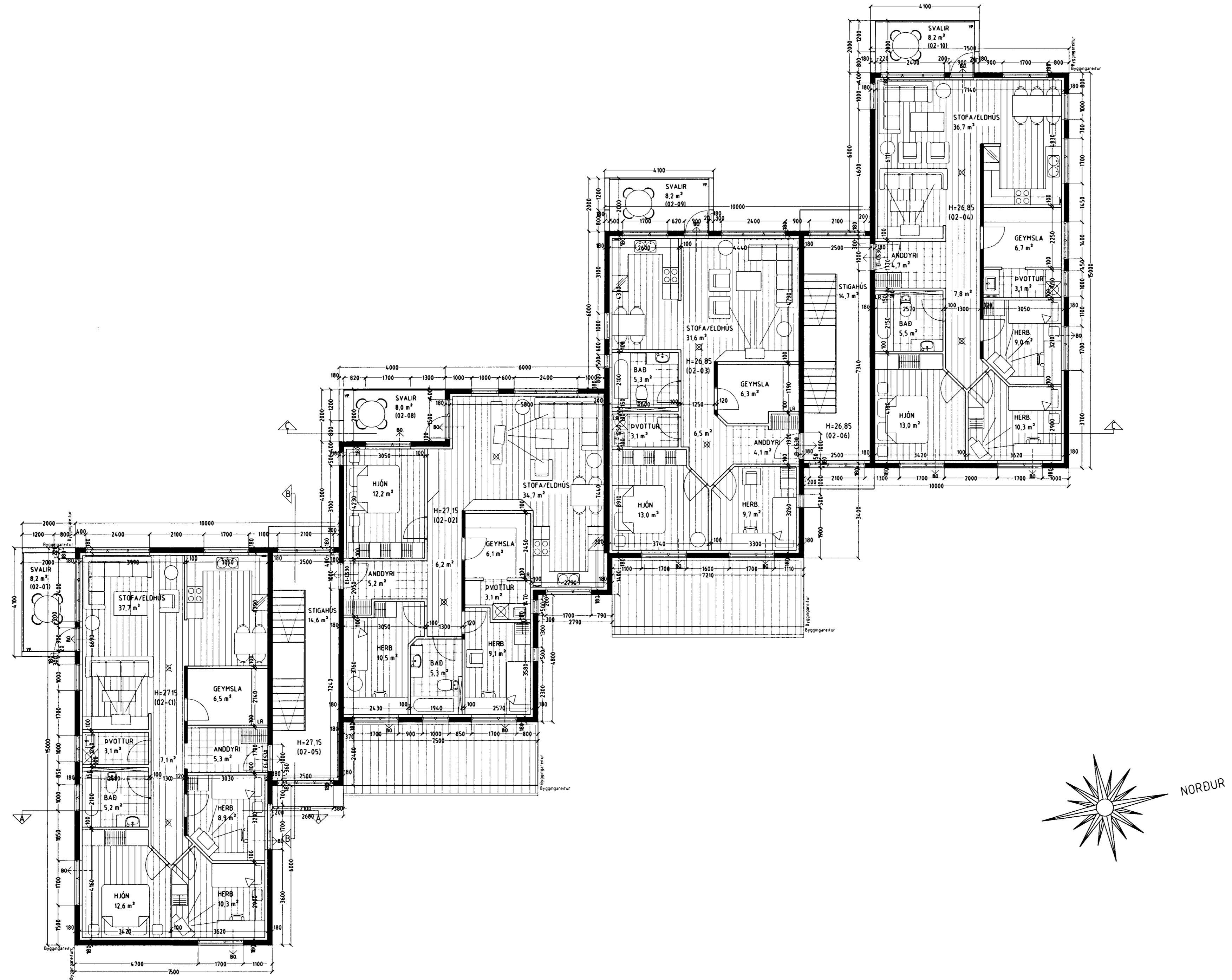
GRUNNMYND 2 HÆÐ. MKV. 1:100.
