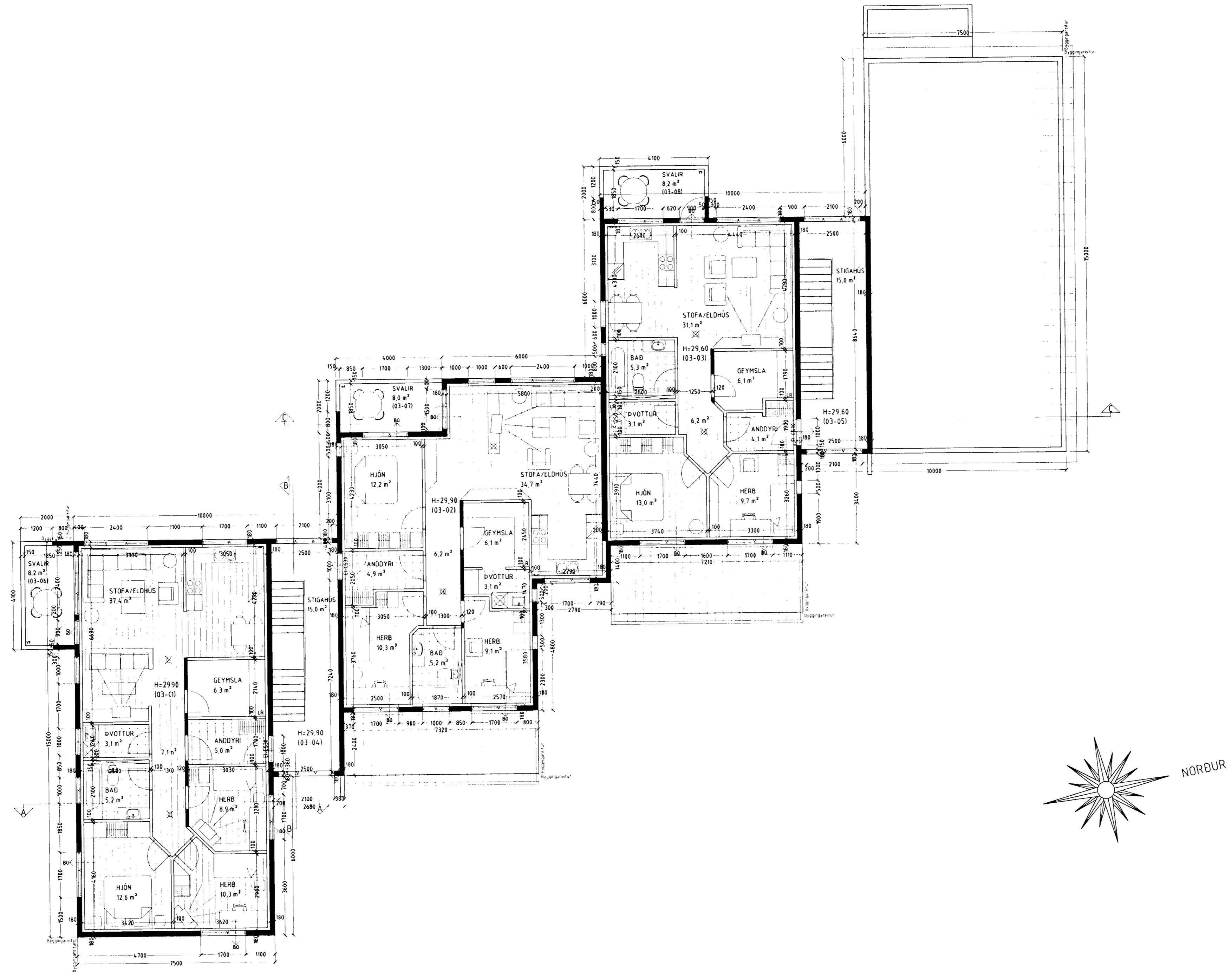
GRUNNMYND 3 HÆÐ. MKV. 1:100.
