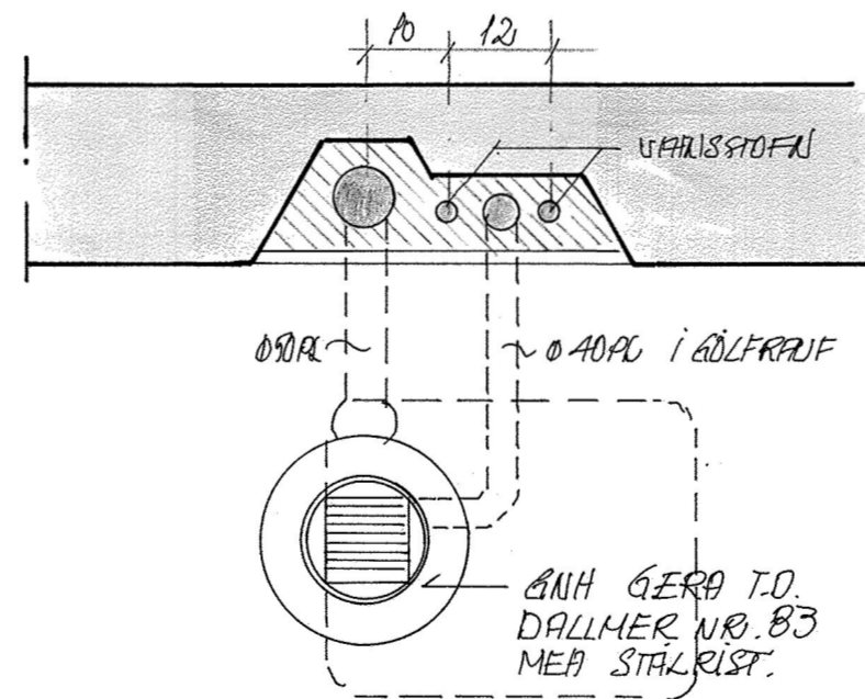
ÞVOTTAH.: GRUNNM. 1:10.
