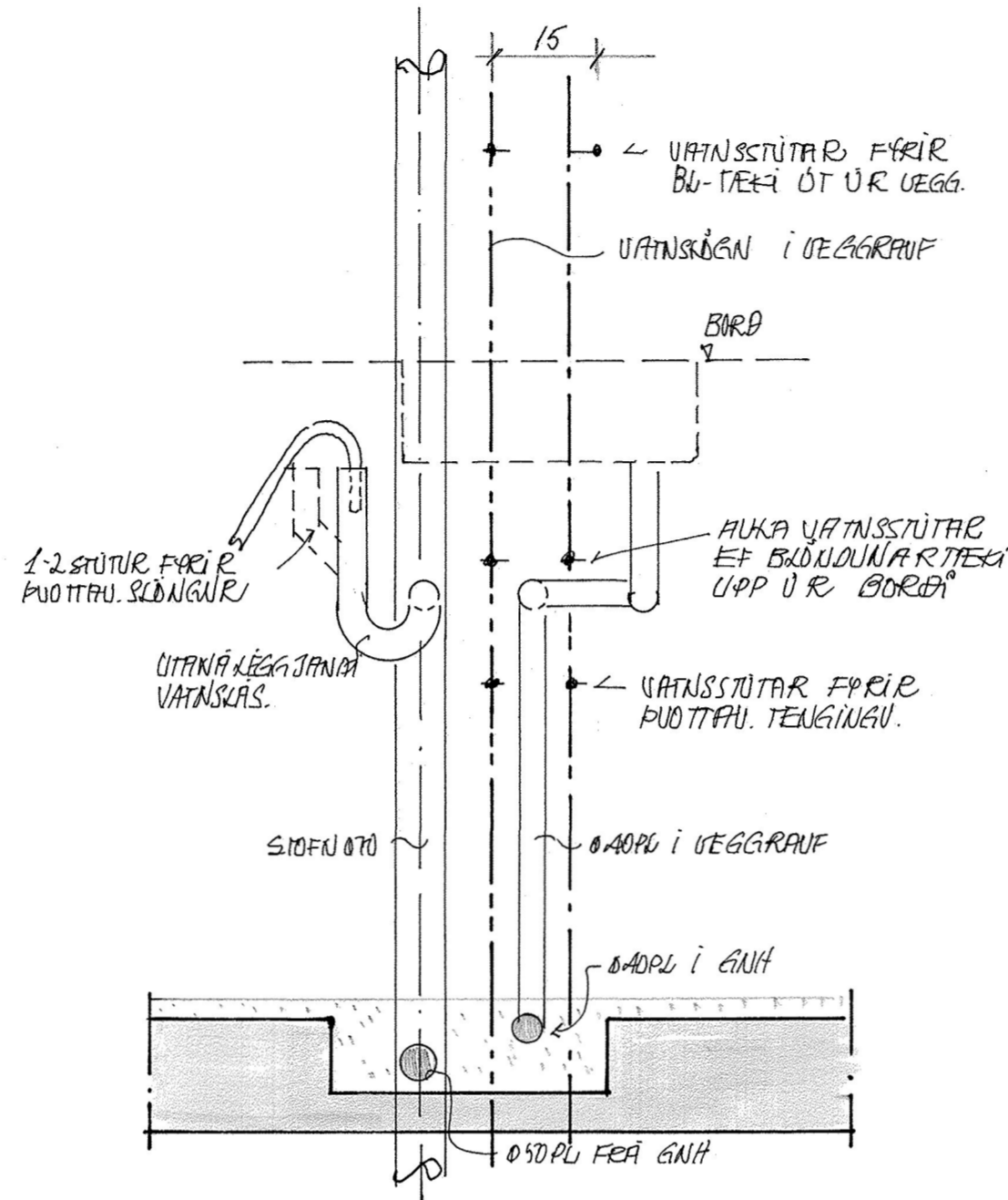
ÞVOTTAH.: GRUNNM. 1:10.
