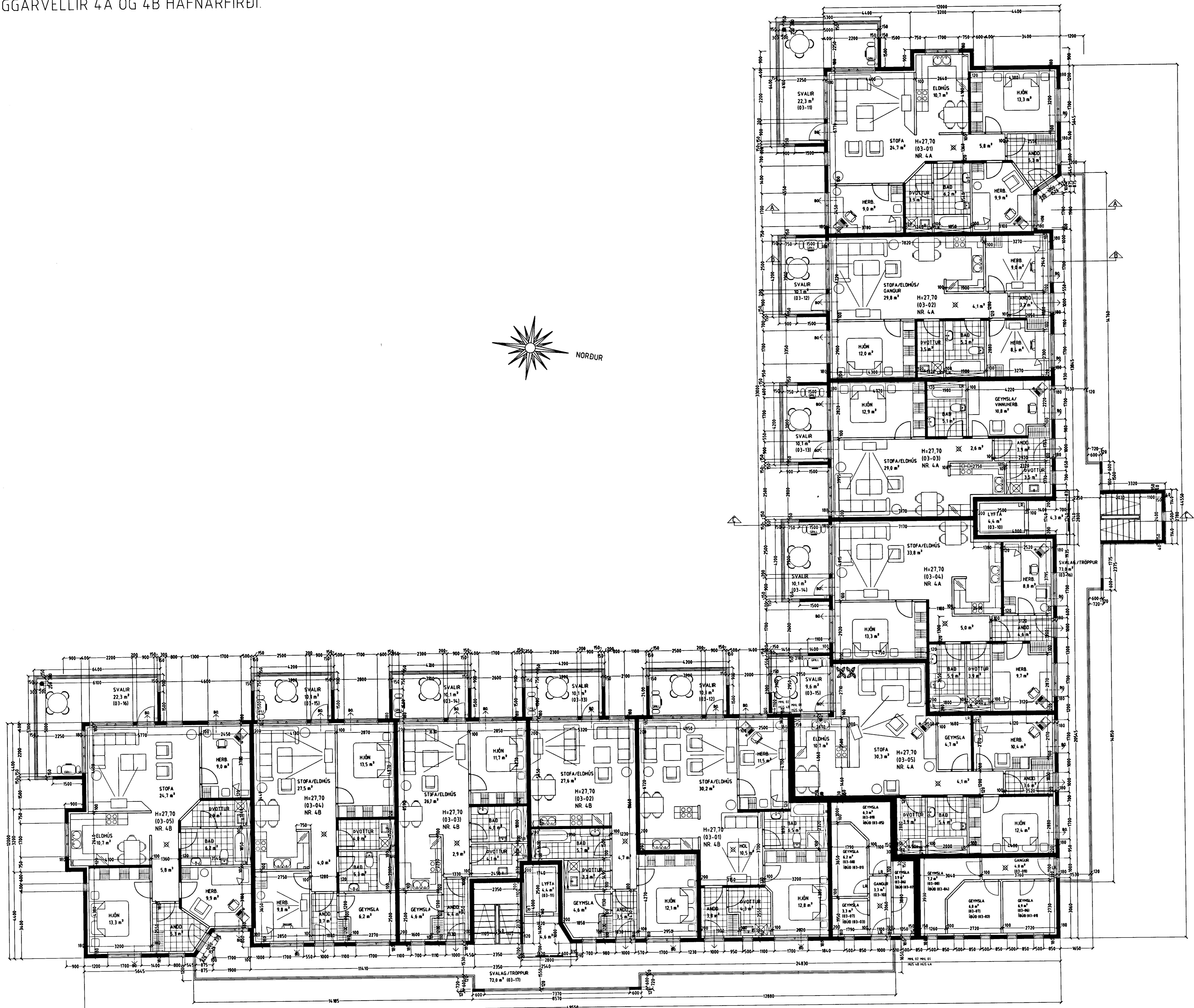
GRUNNMYND 3 HÆÐ MKV. 1:100.
