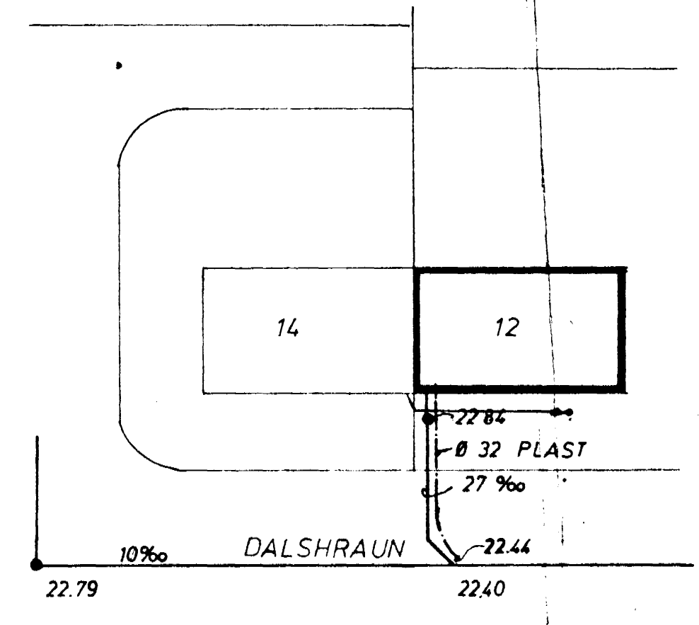
AFSTÖÐUMYND 1:500
