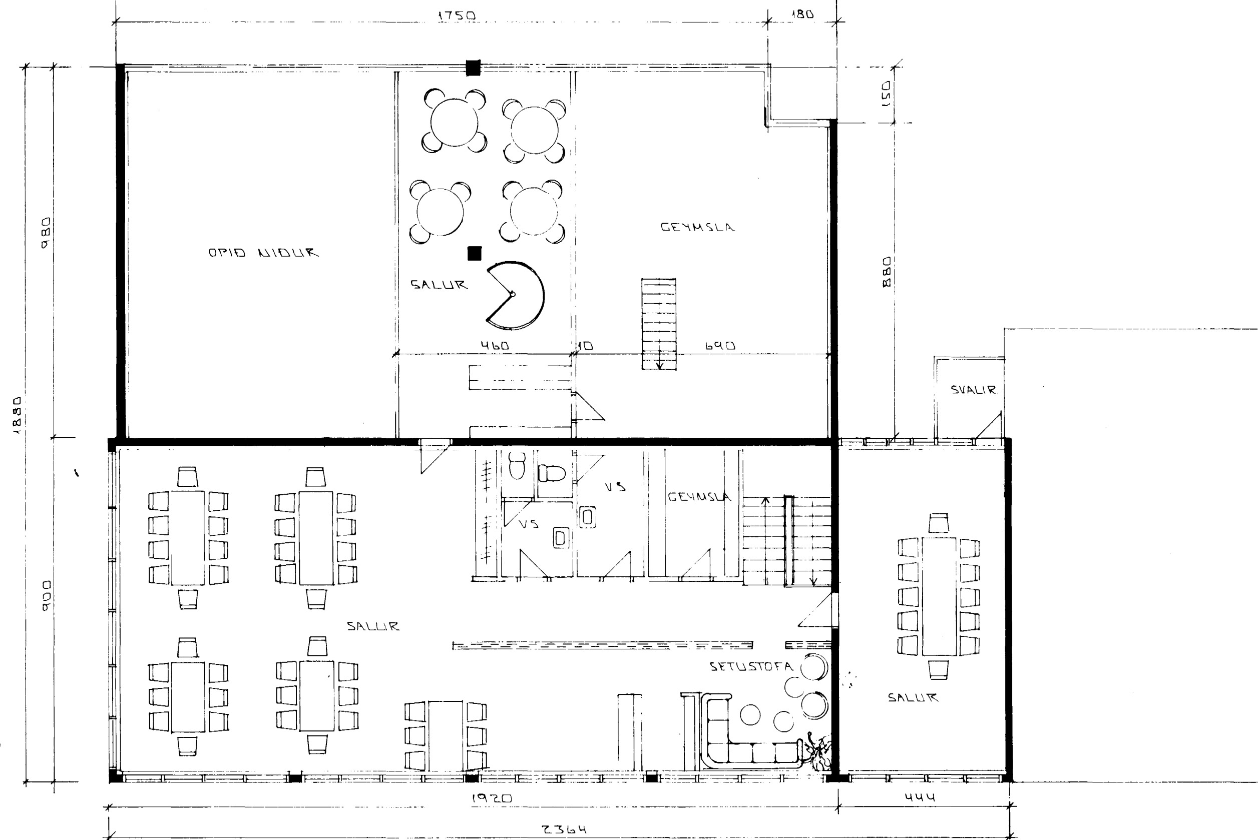
GRUNNMÝND 2. HÆÐAR • 1:100
